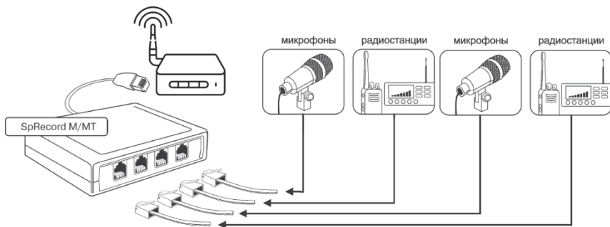
Рисунок 1.1 Система SpRecord
