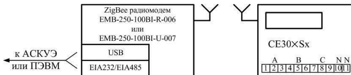
Рисунок 37 – Схема подключения счетчика
