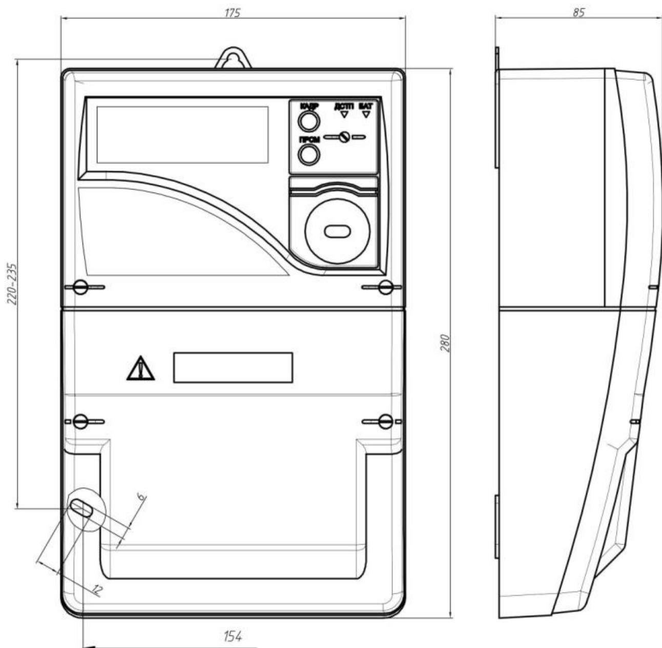
Общий вид счетчика СЕ30х S34
