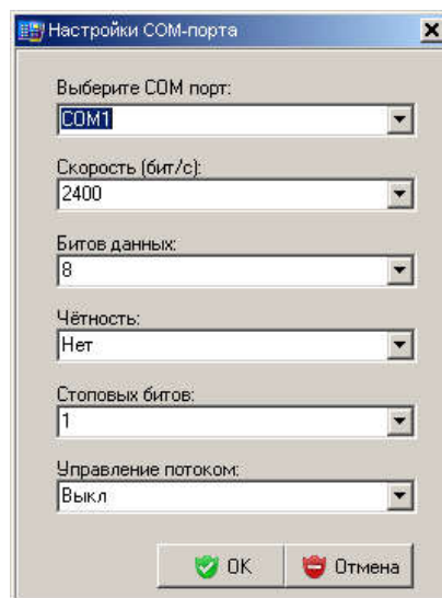
Рисунок 48 – Настройки порта связи PLC-модема CE832C
