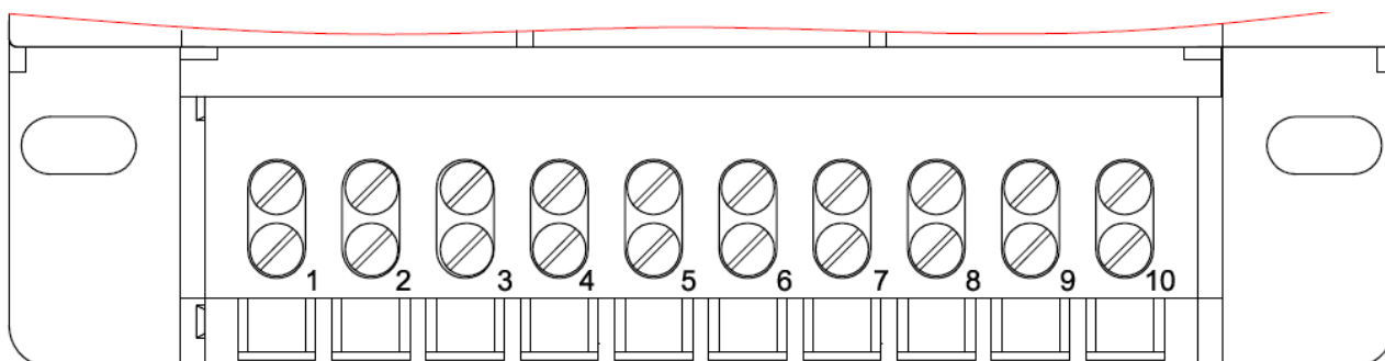
г) – обозначение контактов зажимов счетчика СЕ303 S31 5X3 и СЕ 301 S31 0X3
