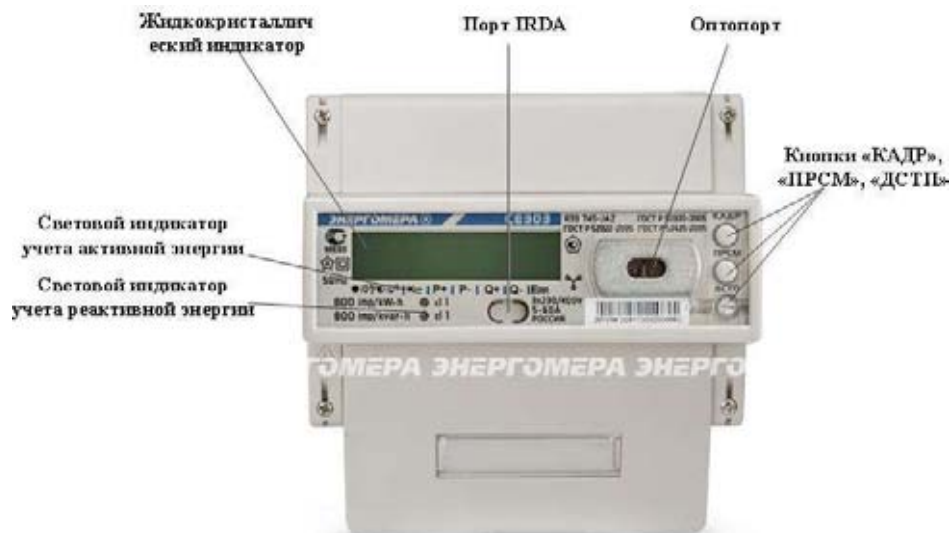
а) CE 303 R33
