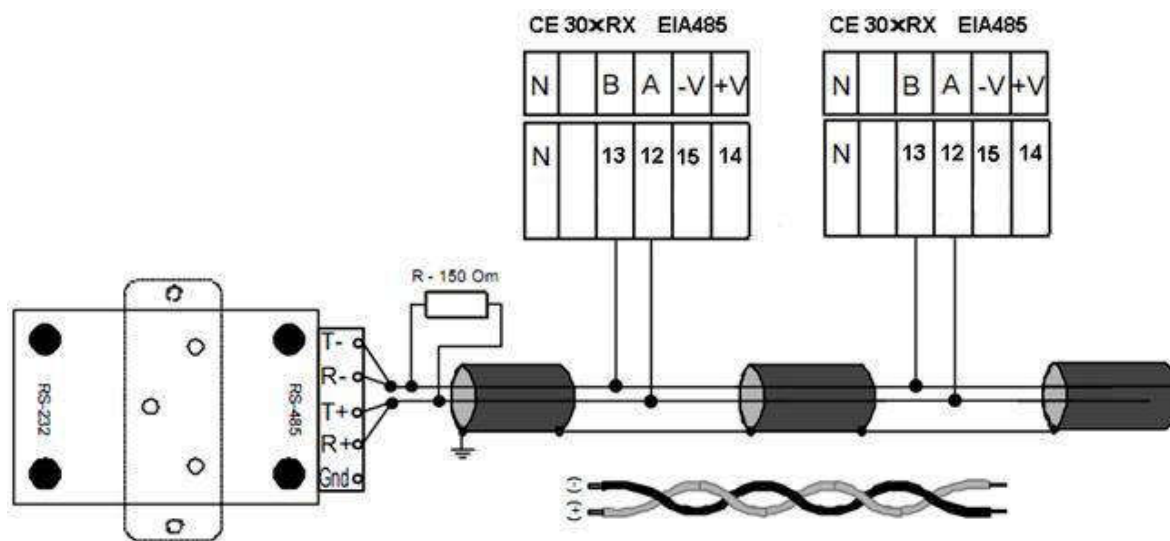
Рисунок 33 – Схема подключения счетчика CE30x R33 с интерфейсом EIA485 через внешний адаптер EIA485/EIA232 к COM-порту ПЭВМ
