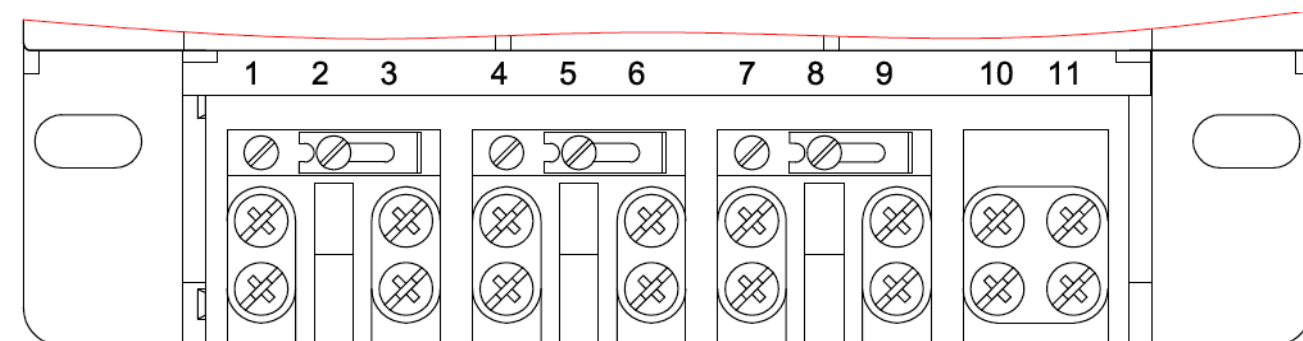
д) – обозначение контактов зажимов счетчика СЕ303 S31 74X и СЕ 301 S31 14X
