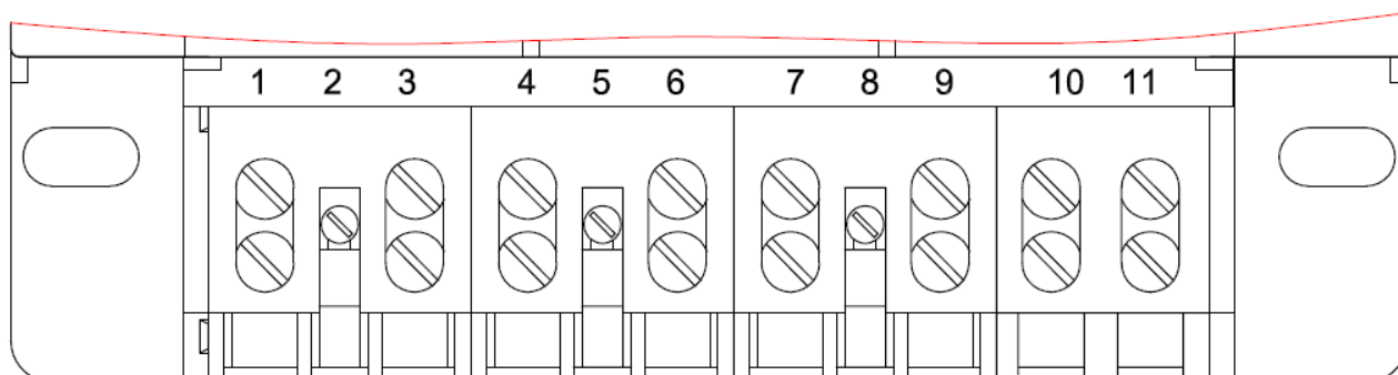
г) – обозначение контактов зажимов счетчика СЕ303 S31 5X3 и СЕ 301 S31 0X3
