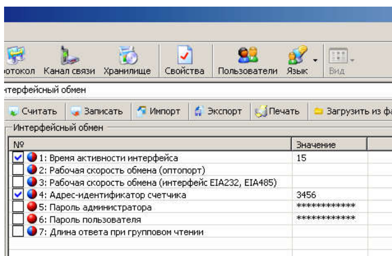
Рисунок 43 – Интерфейсный обмен
