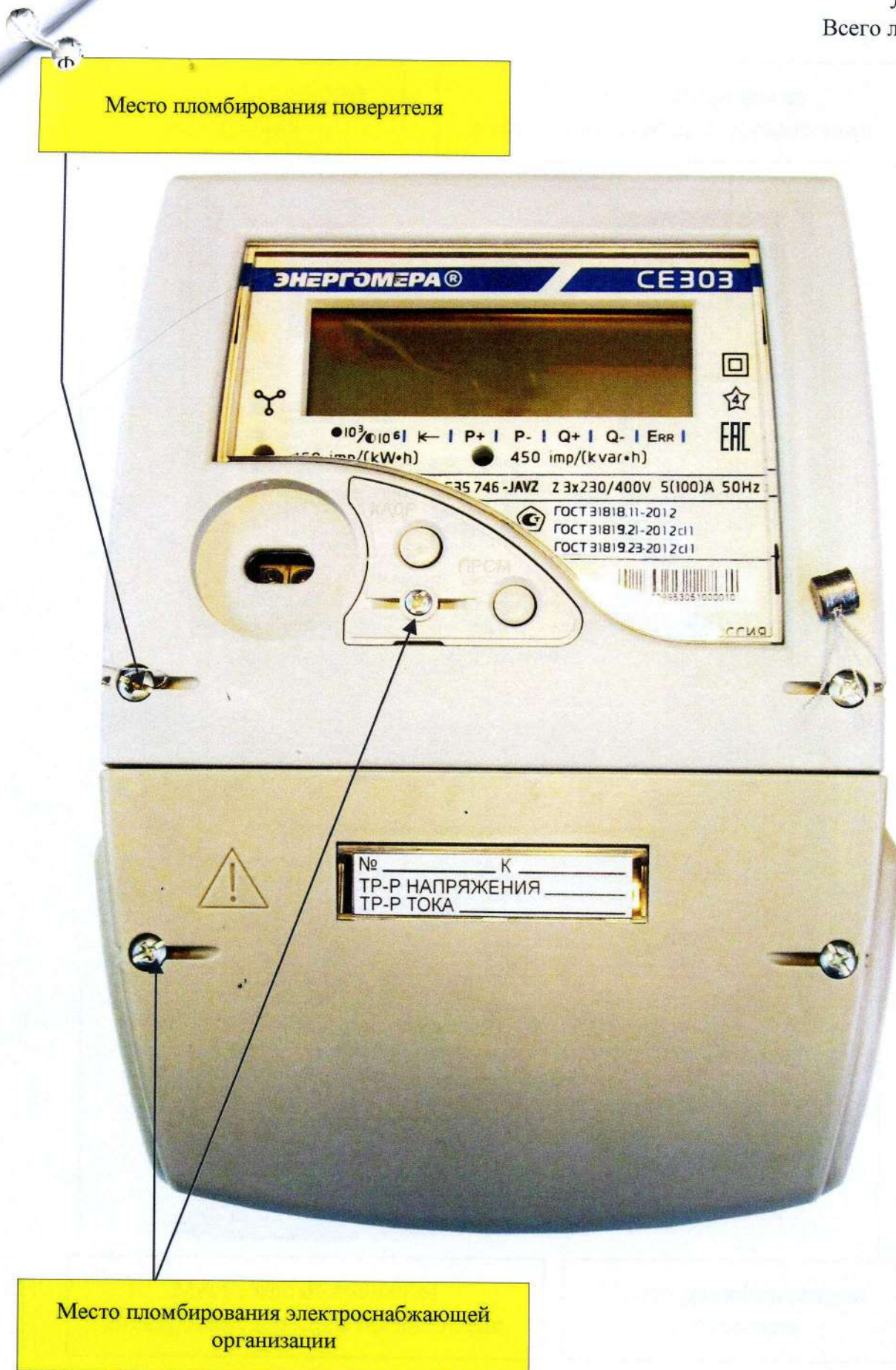
Рисунок 4 - Общий вид счетчика CE 303 S35
