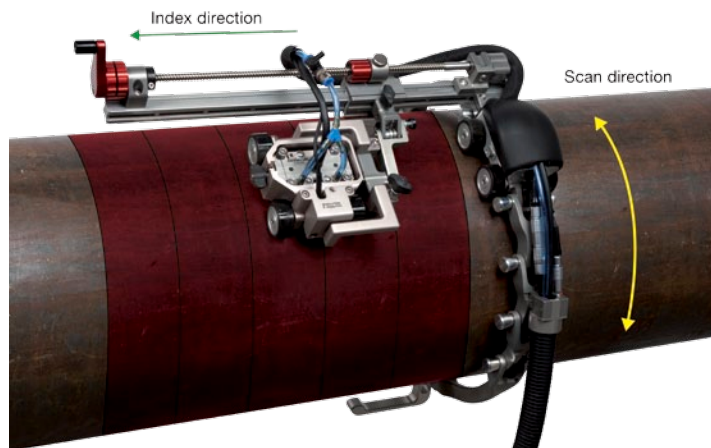
HydroFORM и CHAIN Сканиер
