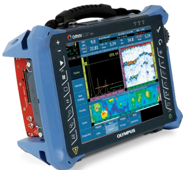
OmniScan MX2 с ФР-модулем 16:128
