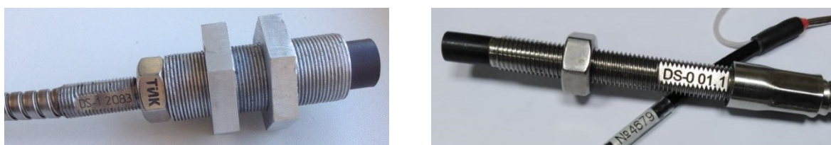
Рисунок 2 – Общий вид вихретоковых преобразователей DS-0, DS-1, DS-2, DS-3
