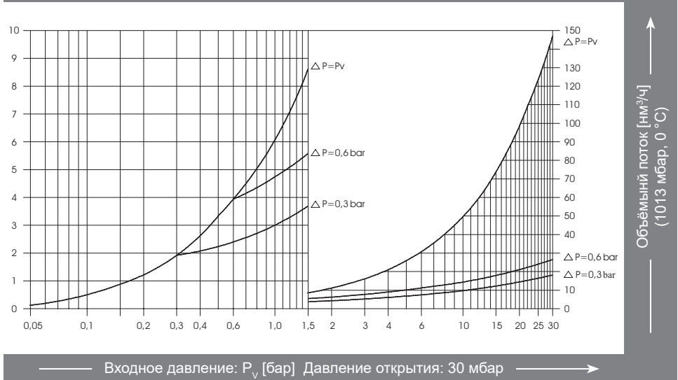
Диаграмма пропускной способности (воздух, 20 °С)
