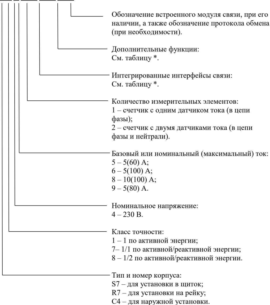
Рисунок 1 - Структура условного обозначения счетчиков
