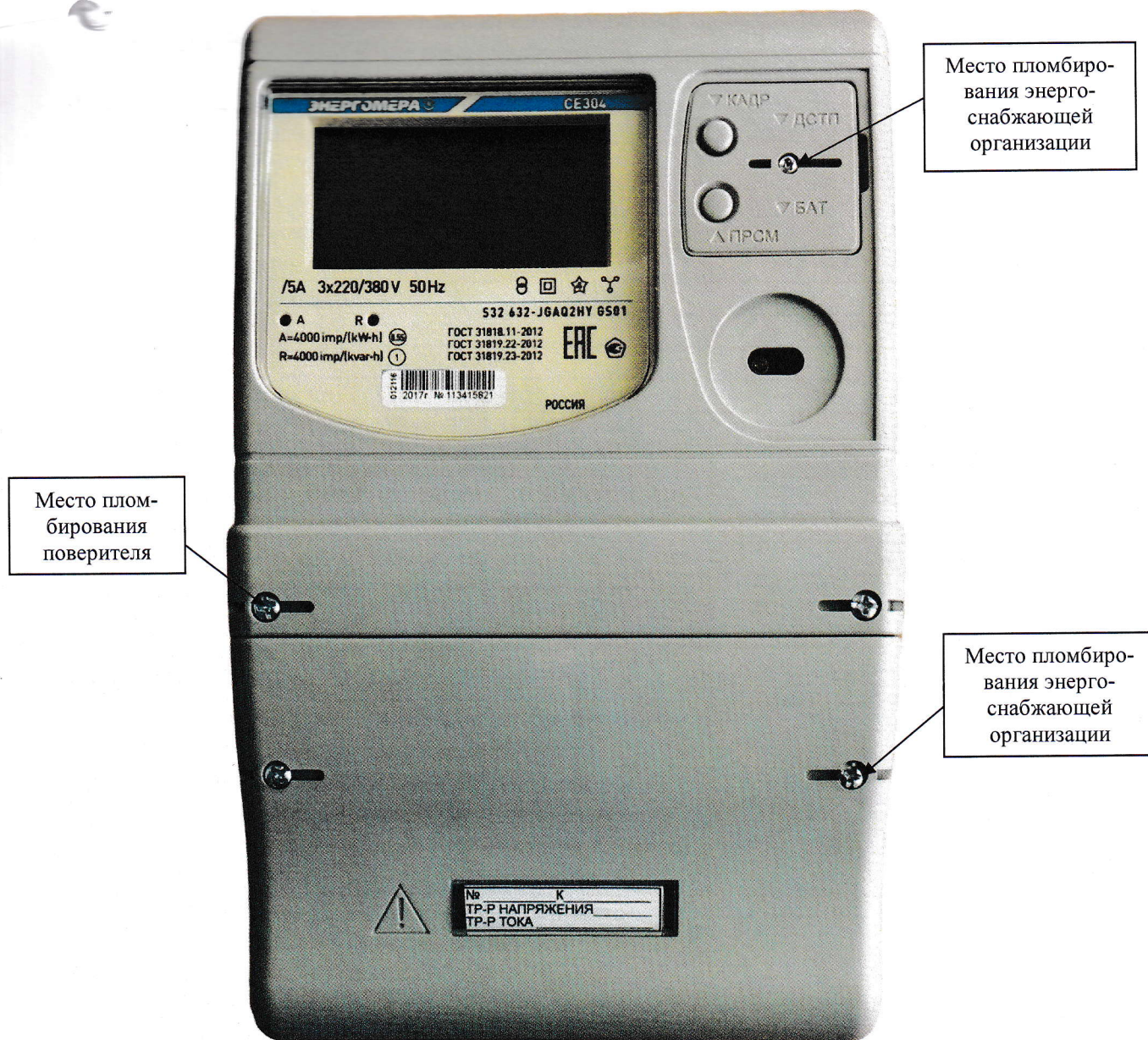
Рисунок 2 – Общий вид счетчика CE 304 S32
