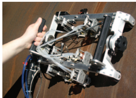
Сканер HSMT-Flex для контроля дифракционно-временным методом (PV-100).
