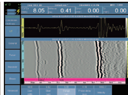
Контроль сварных швов дифракционно-временным методом
