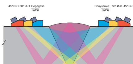
Контроль сварных швов методом TOFD и эхо-импульсным методом.
