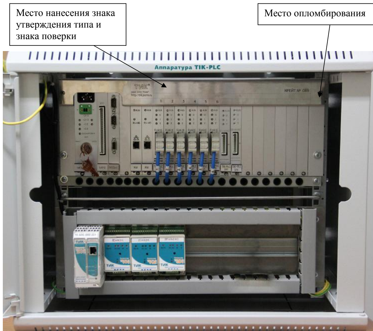
Рисунок 1 – Внешний вид аппаратуры ТИК-PLC
