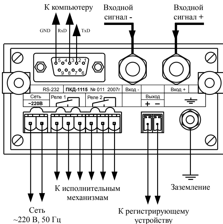
Рисунок Г.2 - Внешние соединения прибора щитового исполнения ПВД-1115.Д
