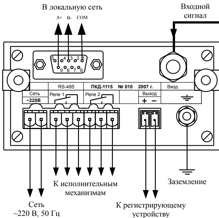
Рисунок Г.1 - Внешние соединения приборов щитового исполнения ПВД-1115.В, ПВД-1115.И, ПВД-1115.ТН
