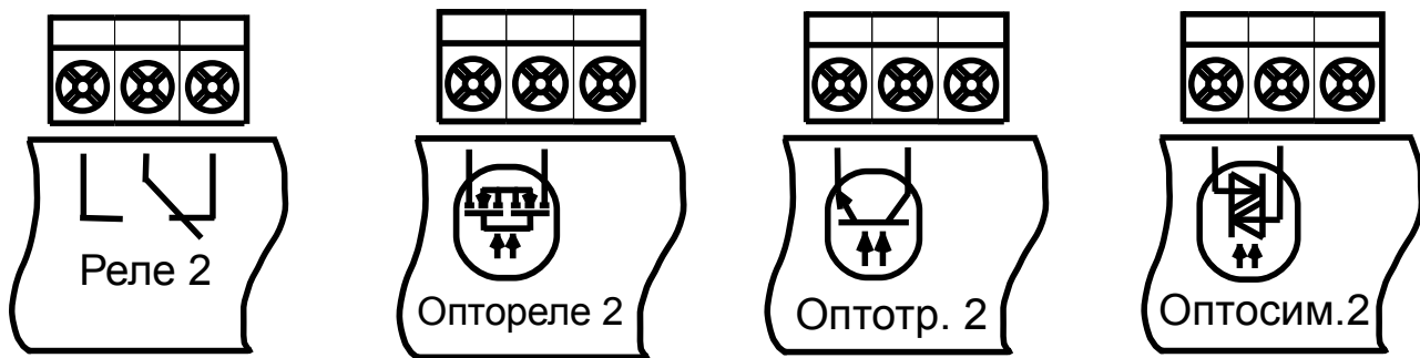
а) электромагнитное реле (сухой контакт)
