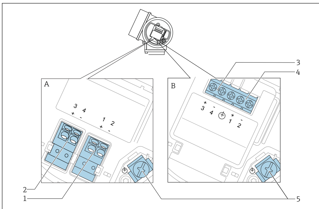
11 Назначение клемм; PROFIBUS PA/FOUNDATION Fieldbus
