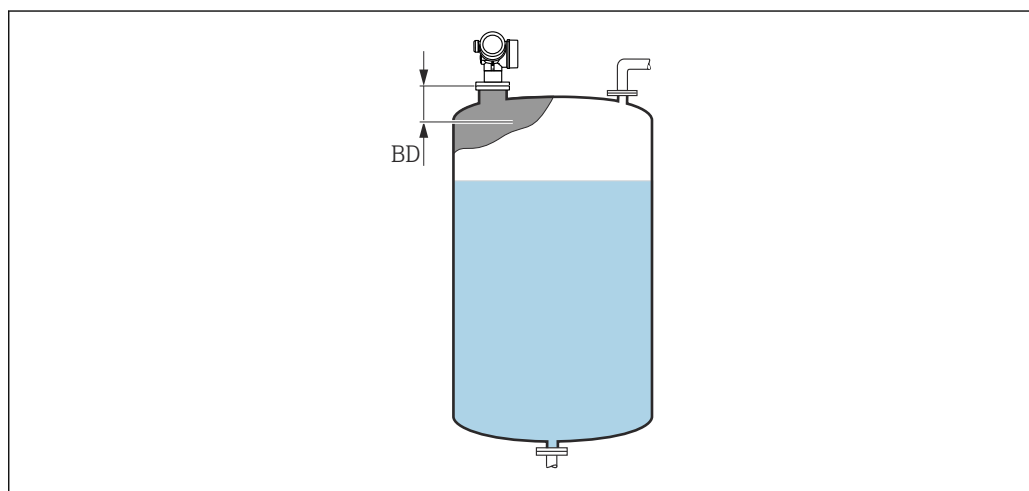
34 Блокирующая дистанция (BD) для измерения в жидких средах
