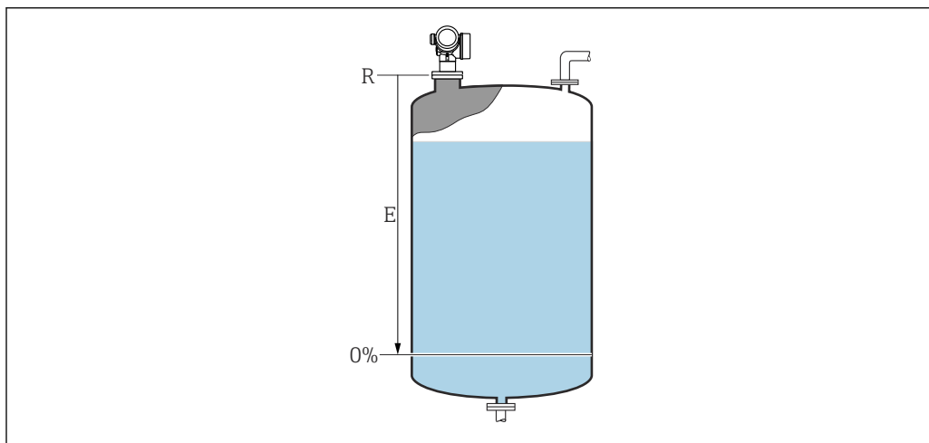
🔗 30 Калибровка пустой емкости (E) для измерения уровня жидких сред A0019486
