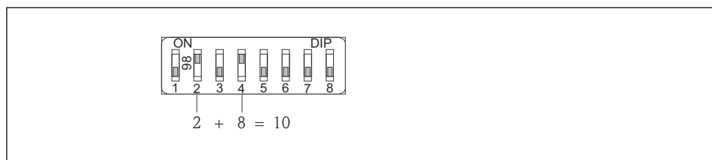
☞ 22 Пример назначения адреса аппаратного средства: переключатель 8 находится в положении «ВЫКЛЮЧЕНО»; переключатели с 1 по 7 определяют адрес.
