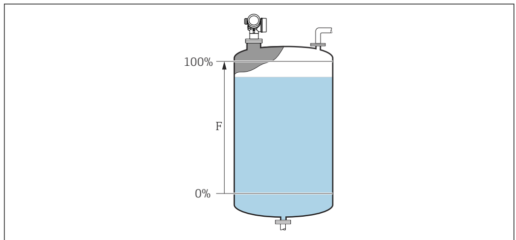
31 Калибровка полной емкости (F) для измерения уровня жидких сред
