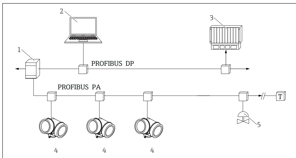
18 Варианты дистанционного управления по протоколу PROFIBUS PA
