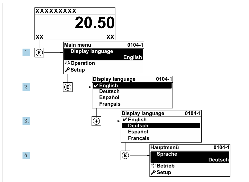
24 Использование примера местного дисплея
