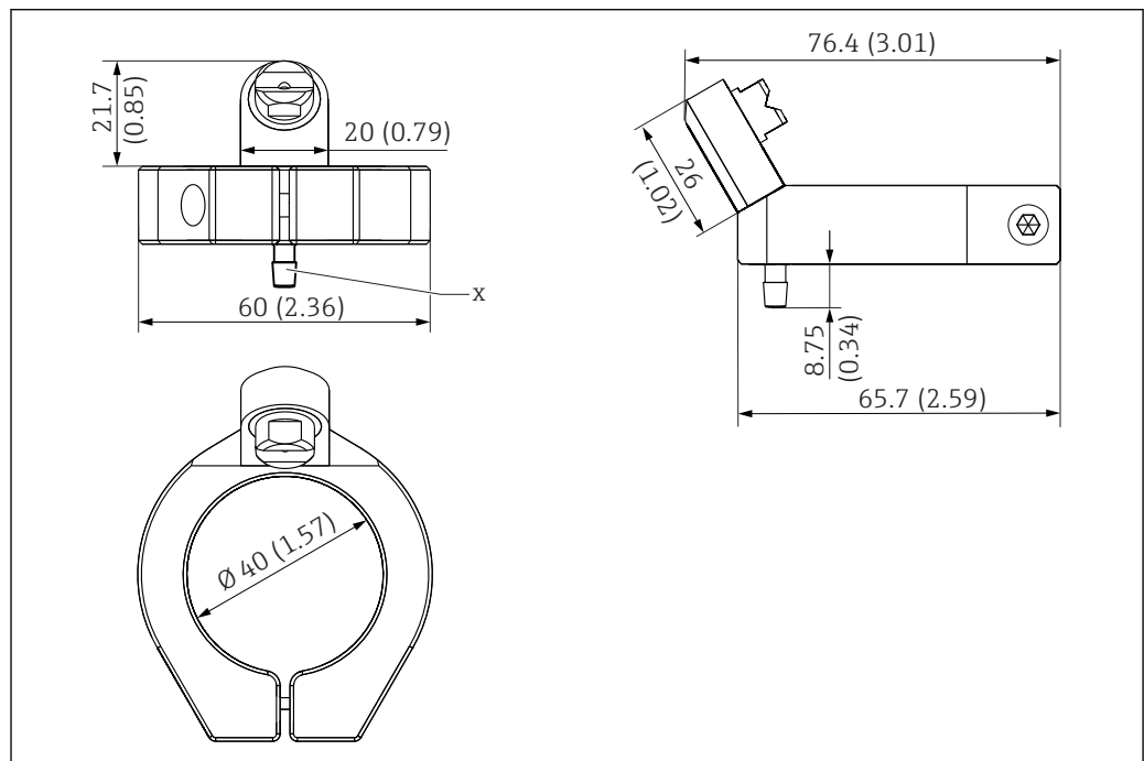
30 Очистка сжатым воздухом для пластикового датчика. Размеры в мм (дюймах)
