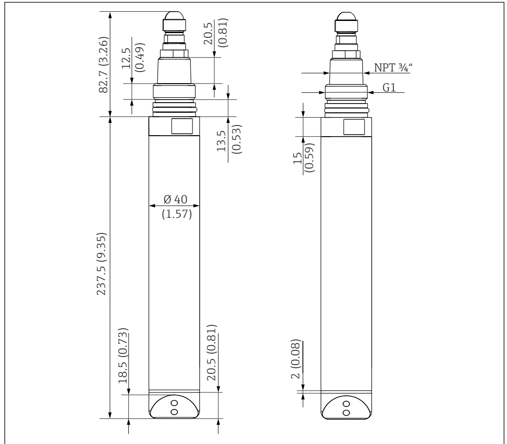
22 Размеры пластмассового датчика. Размеры в мм (дюймах)
