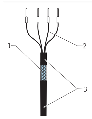
8 Терминированный кабель
