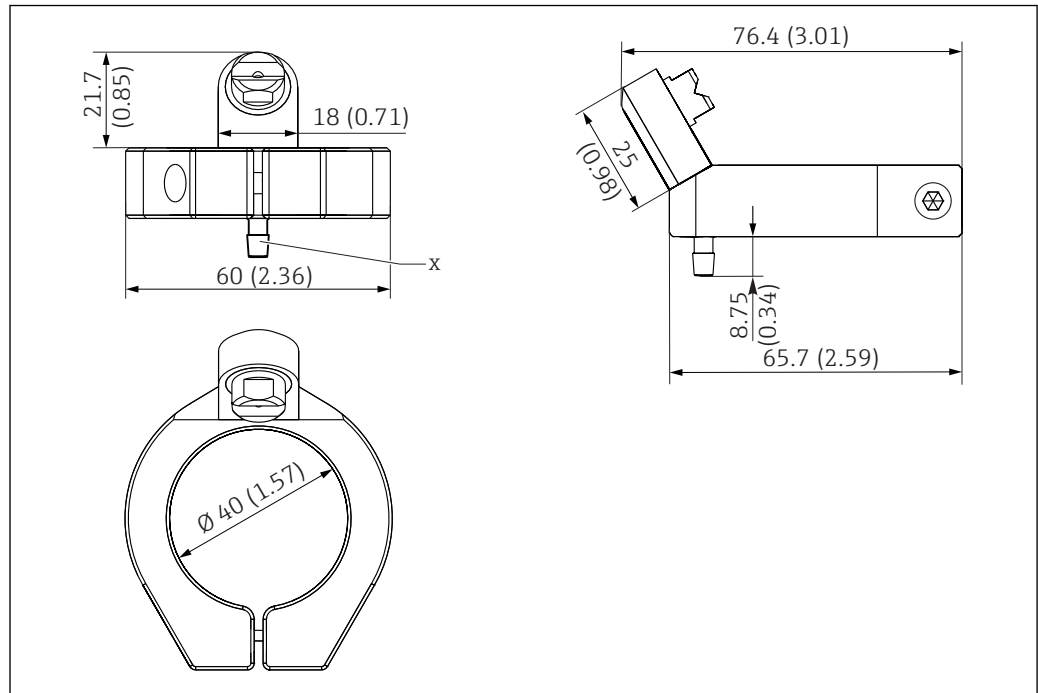
29 Система очистки сжатым воздухом для датчиков из нержавеющей стали. Размеры в мм (дюймах)
