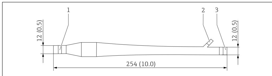
31 Пузырьковая ловушка. Размеры в мм (дюймах)
