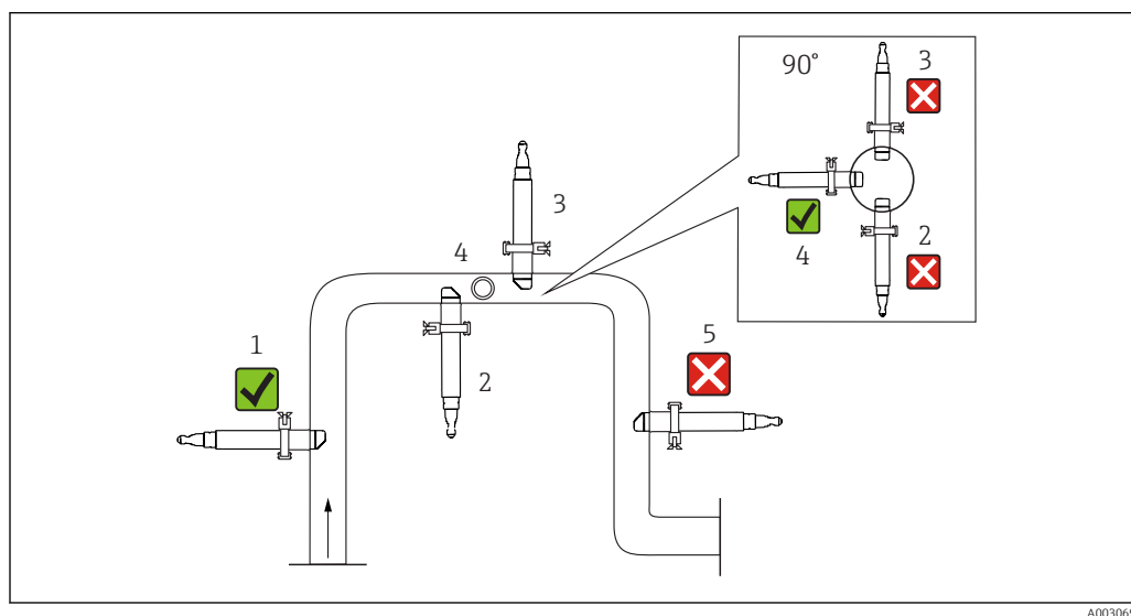
11 Допустимые и неприемлемые варианты ориентации в трубах
