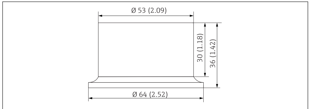
27 Приварной переходник. Размеры в мм (дюймах)
