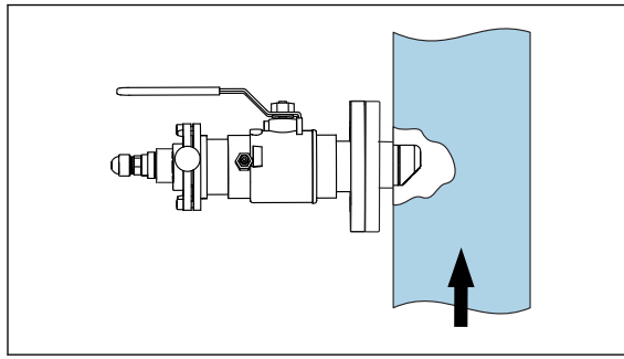
14 Монтаж с выдвижной арматурой CUA451
