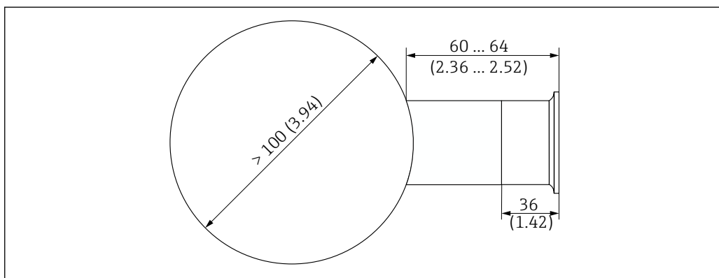
21 Трубное соединение с приварным переходником. Размеры в мм (дюймах)
