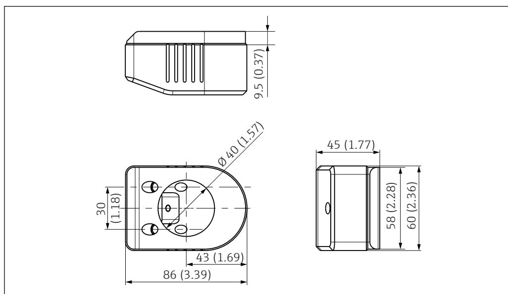
26 Полупроводниковый эталон Calkit CUS52D. Размеры в мм (дюймах)
