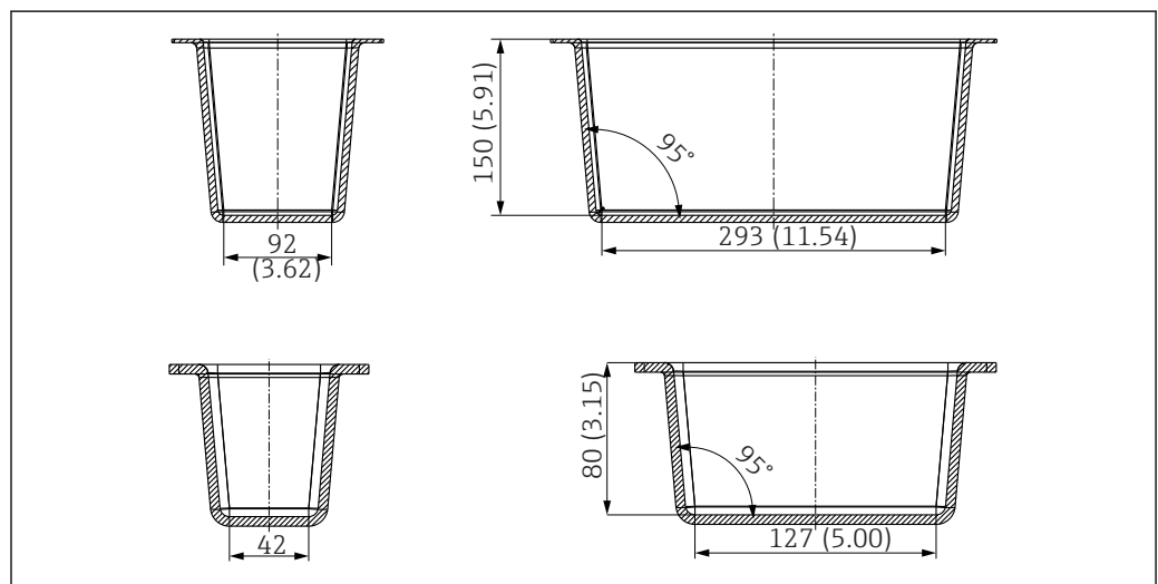
6 Большой калибровочный резервуар (вверху) и малый калибровочный резервуар (внизу). Размеры в мм (дюймах)
