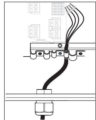
10 Затягивание винта
