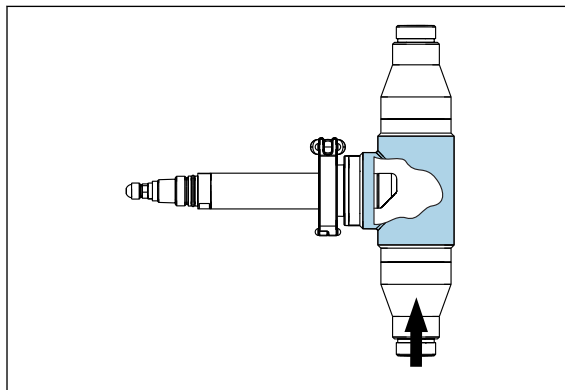
17 Монтаж с проточной арматурой CUA252
