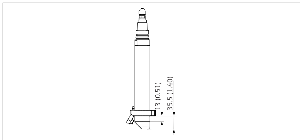
25 Размеры датчика с системой очистки сжатым воздухом. Размеры в мм (дюймах)
