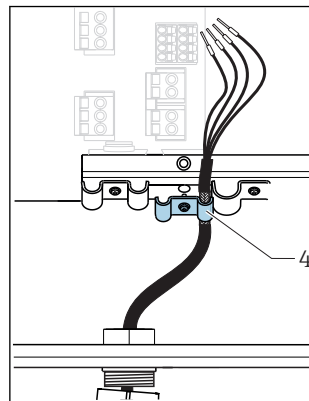
9 Вставка кабеля
