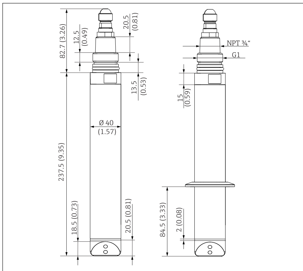
23 Размеры датчика из нержавеющей стали и датчика из нержавеющей стали с зажимным соединением (справа). Размеры в мм (дюймах)
