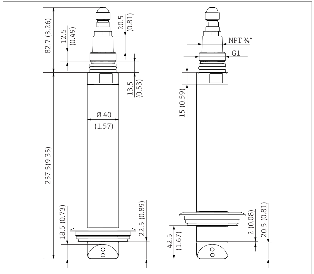
24 Размеры датчика из нержавеющей стали со стандартным соединением Varivent (слева) и удлиненным стержнем (справа). Размеры в мм (дюймах)
