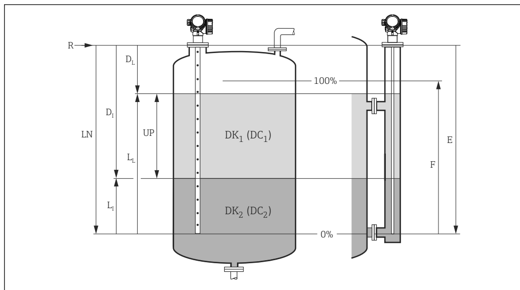
22 Параметры конфигурации измерения уровня границы раздела фаз
