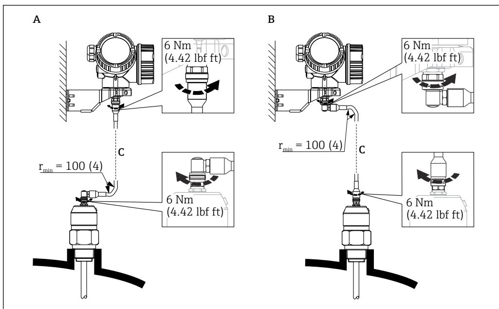
7 Подключение кабеля. Варианты
