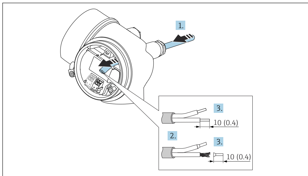
13 Размеры: мм (дюймы)
