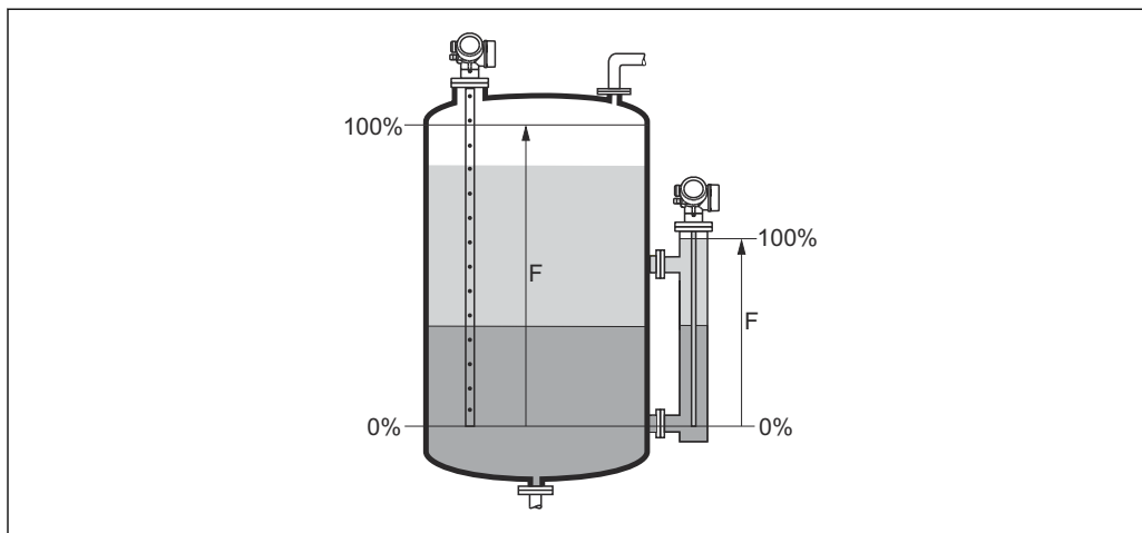
33 Калибровка полной емкости (F) для измерения уровня границы раздела фаз
