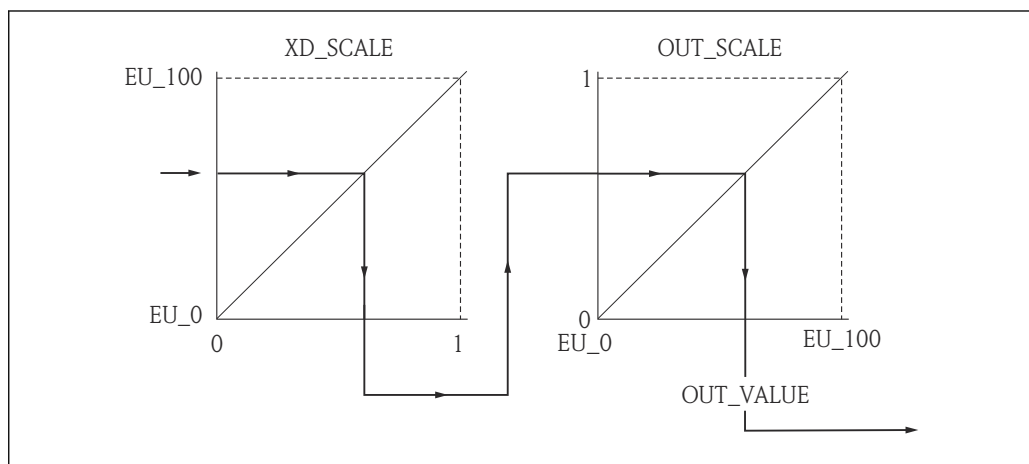
24 Масштабирование измеренного значения в блоке AI
