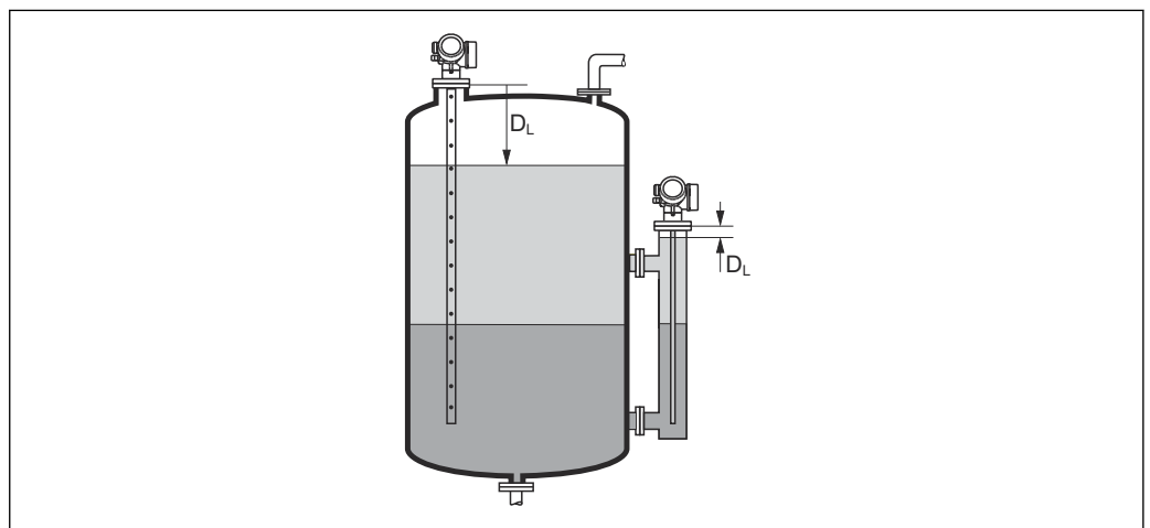
35 Расстояние для измерения уровня границы раздела фаз
