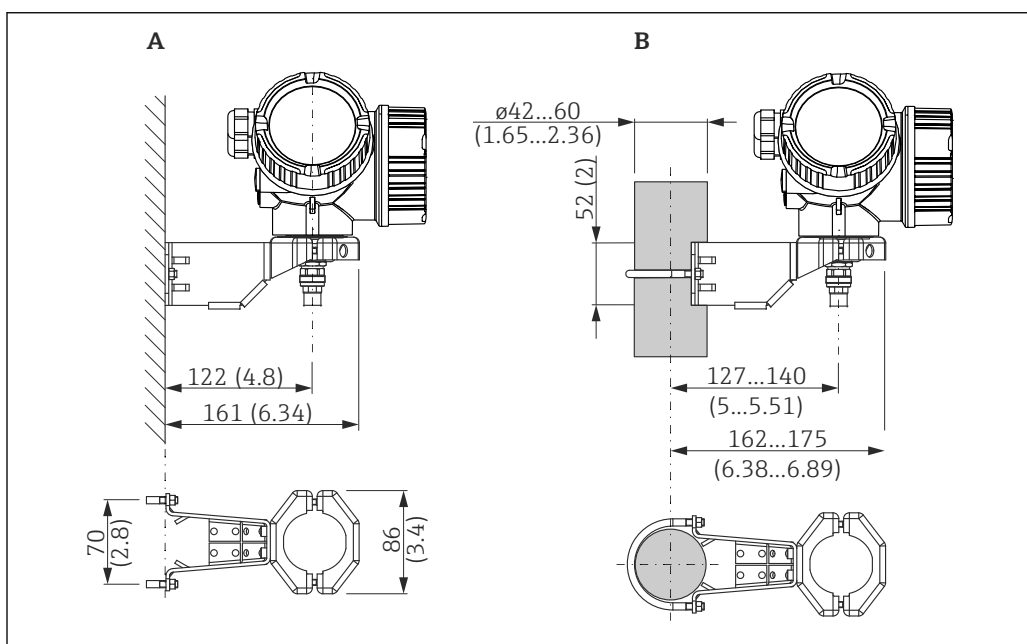
6 Монтаж корпуса электронной части с использованием кронштейна; размеры: мм (дюйм)
