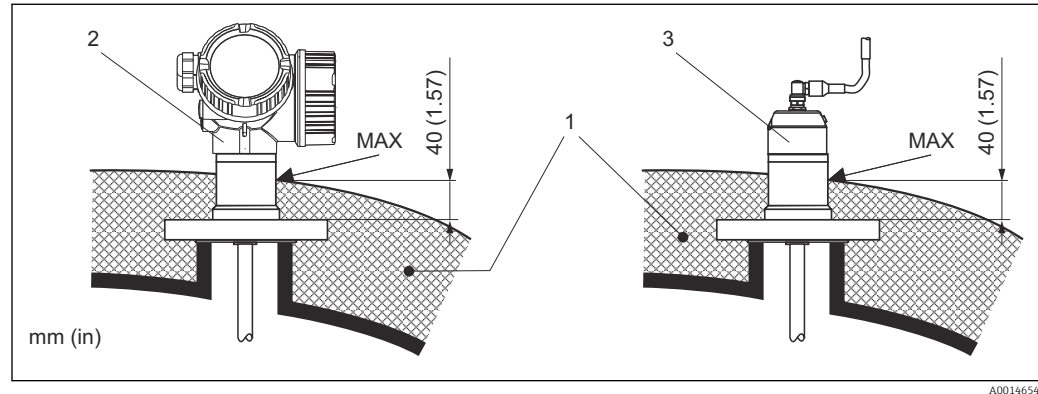
5 Фланцевое присоединение к процессу – FMP55
