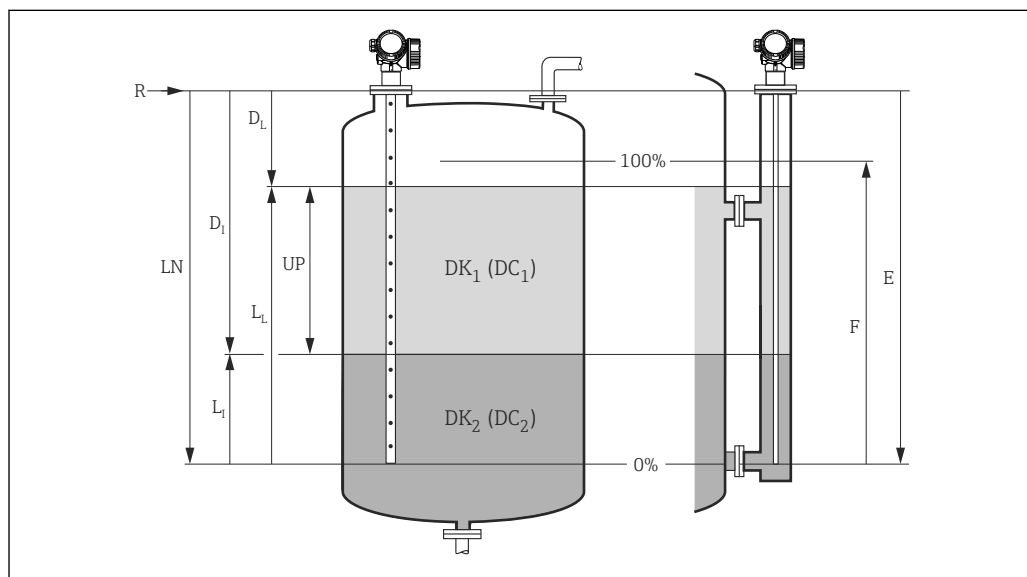
25 Параметры конфигурации измерения границы раздела фаз
