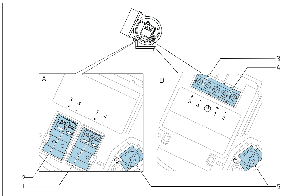
9 Назначение клемм; PROFIBUS PA/FOUNDATION Fieldbus
