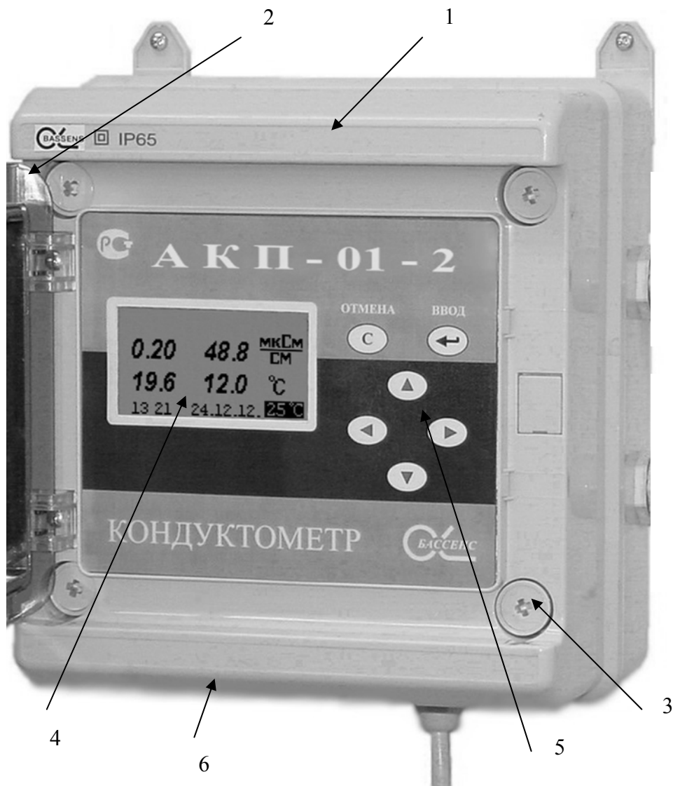
Рис. 1.4.3-1 Измерительное устройство анализатора АКП-01-2К.
