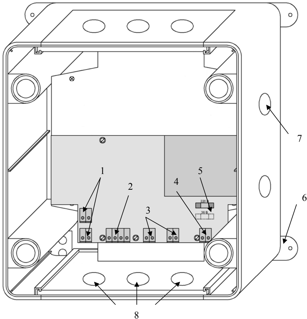
Рис.2.2.1-2 Нижний отсек измерительного устройства
