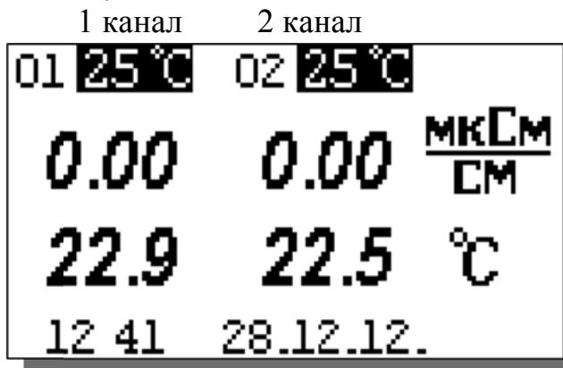
Рис. 2.3.1-2. Окно измерений АКП-01-2К для двух каналов
