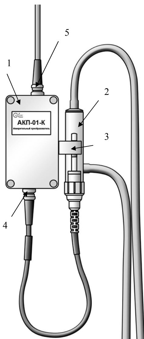
Рис. 1.4-1-1 Измерительный преобразователь анализатора АКП-01-2К.
