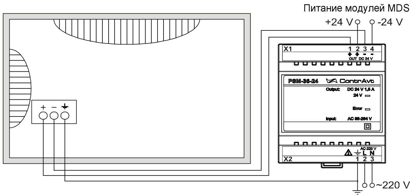
Рисунок 5 – Подключение электропитания
