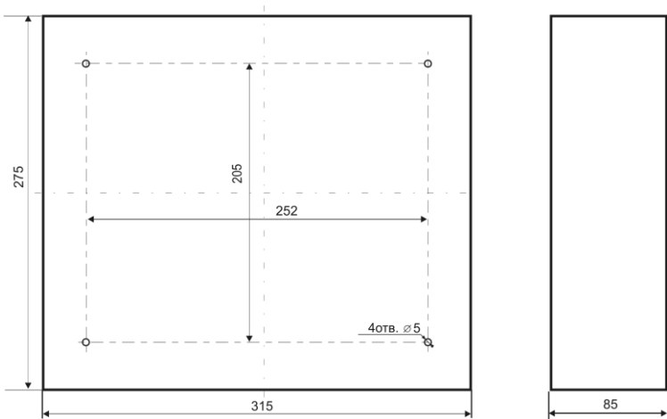
Рис.3 Установочные размеры БПР24-100 исп.1
