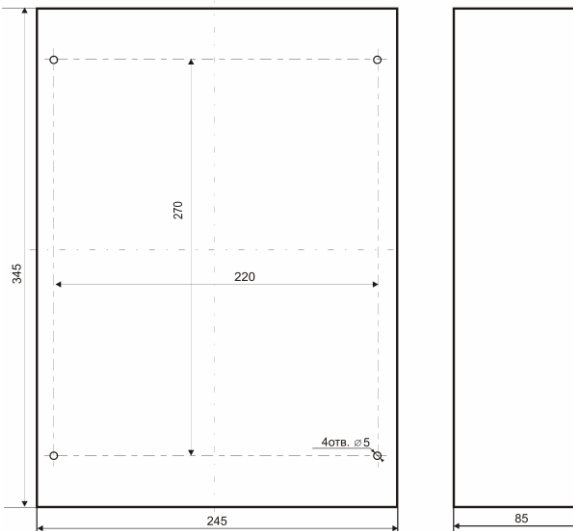
Рис.2 Установочные размеры БПР12-100 исп.1
