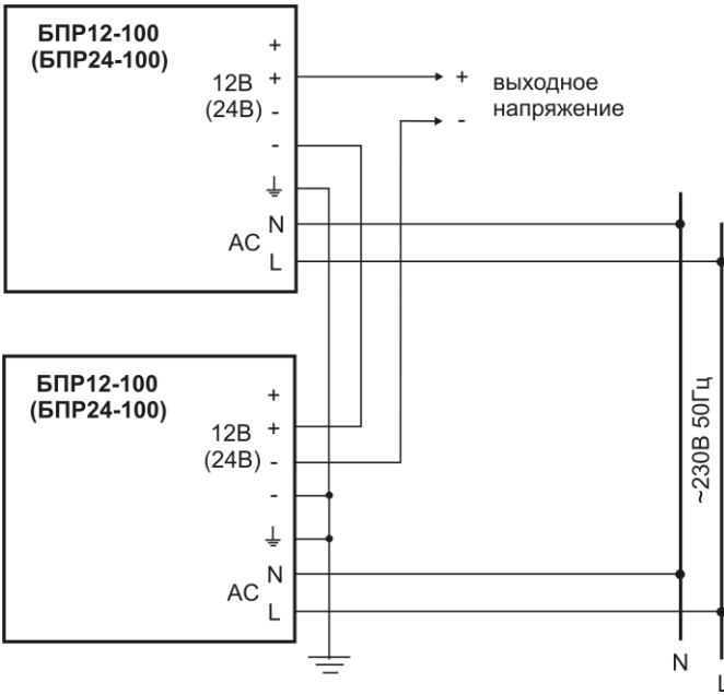
Рис.5 Последовательное включение БПР для увеличения выходного напряжения
