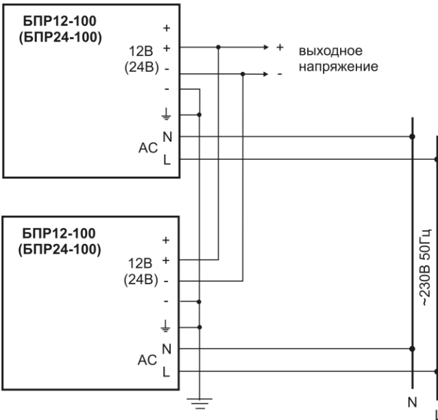
Рис.6 Параллельное включение БПР для увеличения выходного тока
