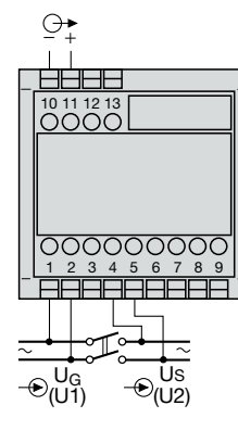
Fig. 3. Alimenté interne par l'entrée de mesure, alimentation auxiliaire pas nécessaire.
