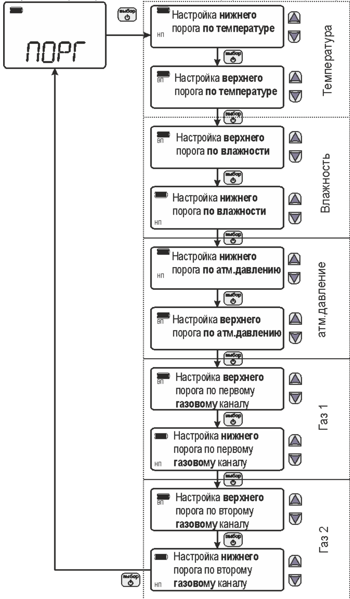
Рисунок 5.9 Установка порогов
