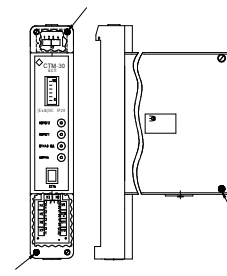
Рисунок 2н - БСП сигнализаторов STM-30-54...STM-30-57
