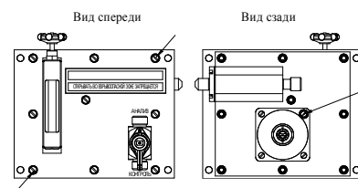
Рисунок 2в - БД сигнализаторов STM-30-07
