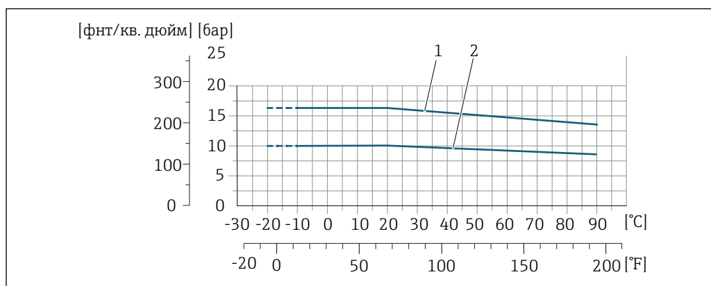
35 Материал присоединения к процессу: нержавеющая сталь (-20 °C (-4 °F)); углеродистая сталь (-10 °C (14 °F))
