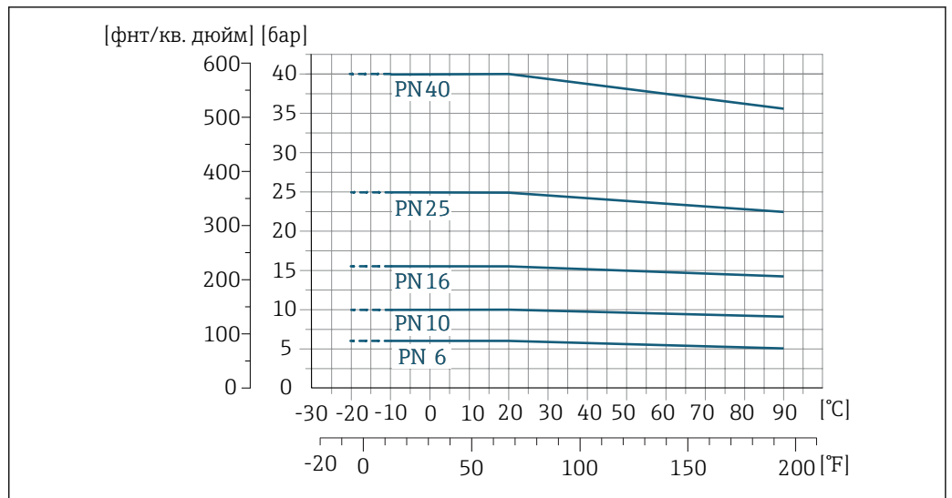
28 Материал присоединения к процессу: нержавеющая сталь (-20 °C (-4 °F)); углеродистая сталь (-10 °C (14 °F))
