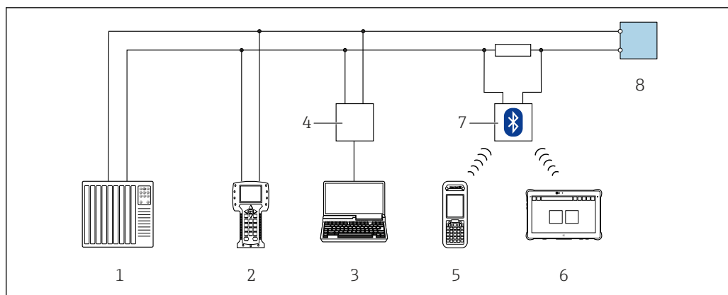
46 Варианты дистанционного управления по протоколу HART (активный режим)
