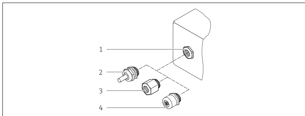
43 Доступные кабельные вводы и уплотнения
