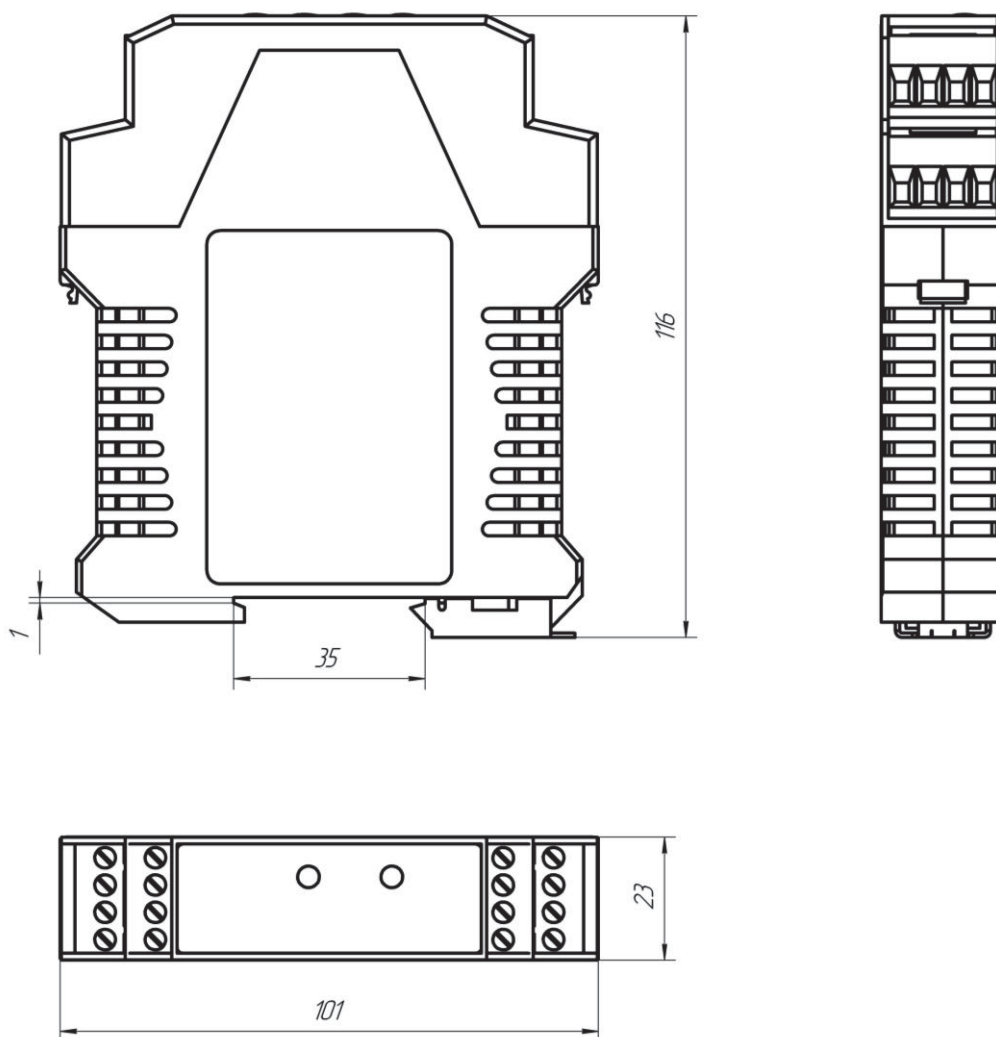
Рисунок Б.1 – Габаритные размеры Источника ЭЛМЕТРО – ИПТ – 2, не более.
