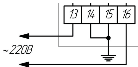
Рисунок В.1 – Схема подключения ЭЛМЕТРО – ИПТ – 2.
