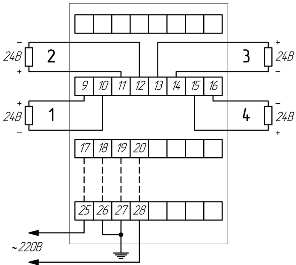
Рисунок В.2 – Схема подключения ЭЛМЕТРО – ИПТ – 4.
