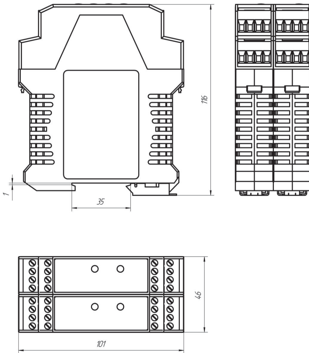
Рисунок Б.2 – Габаритные размеры Источника ЭЛМЕТРО – ИПТ – 4, не более.
