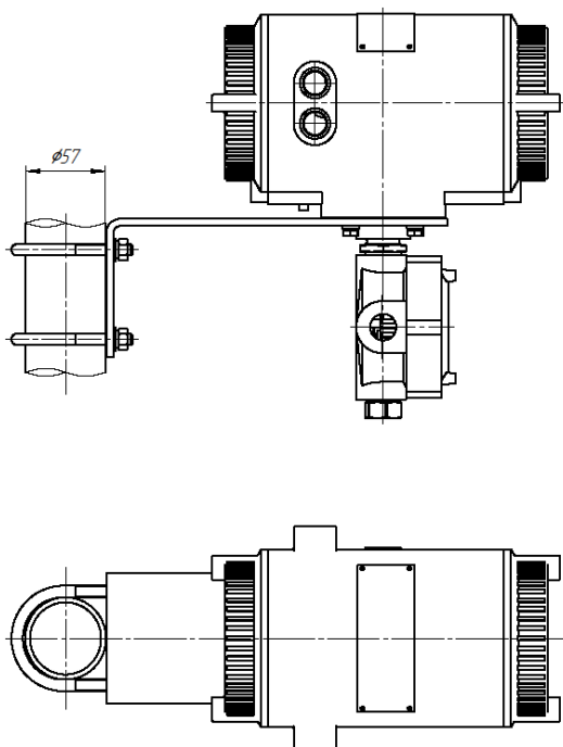
Рисунок А.13 – Комплект монтажа электронного блока расширенного исполнения, дистанционного расходомера ЭМИС-МАСС 260
