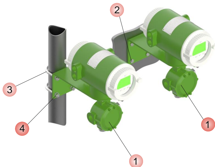
Рисунок 2.8 – Варианты установки электронного блока дистанционного расходомера
