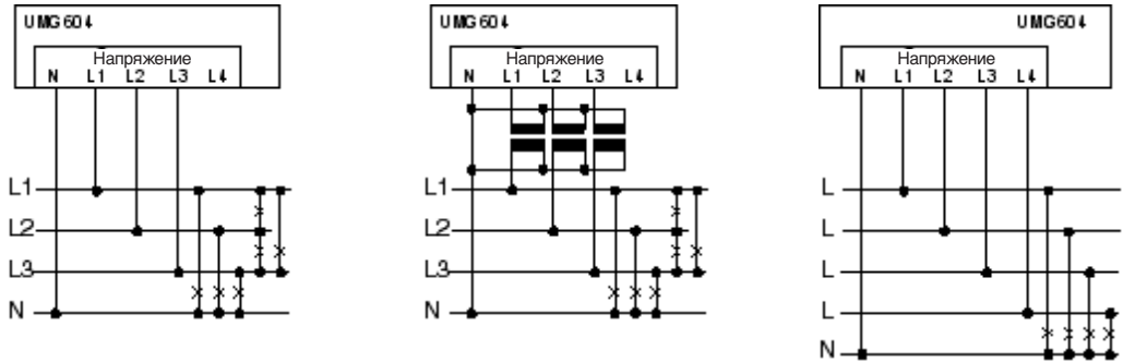
Рис. 31.1. Примеры подключения для измерения напряжения в "трехфазных 4-проводных сетях". (Пример подключения 0, см. стр. 51)
