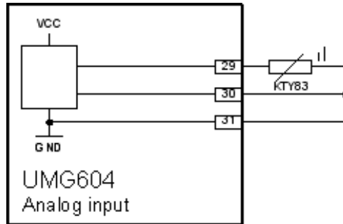
Рис. 42.1. Пример, измерение температуры при помощи КТУ83.
