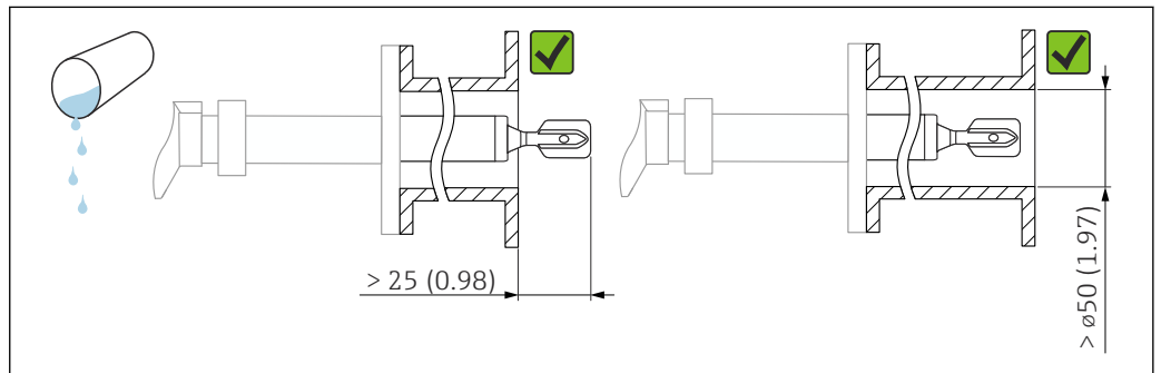
8 Пример монтажа для жидкостей с низкой вязкостью. Единица измерения мм (дюйм)
