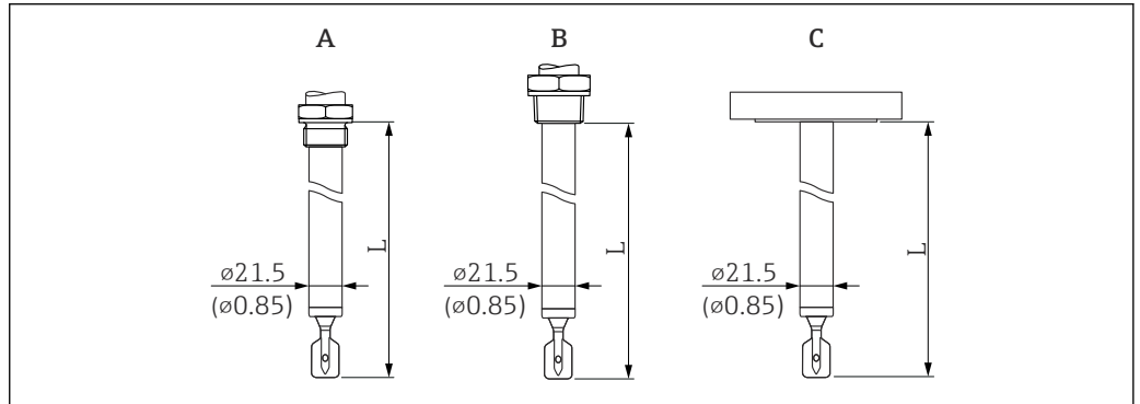
20 Удлинительная трубка, длина датчика L. Единица измерения мм (дюйм)
