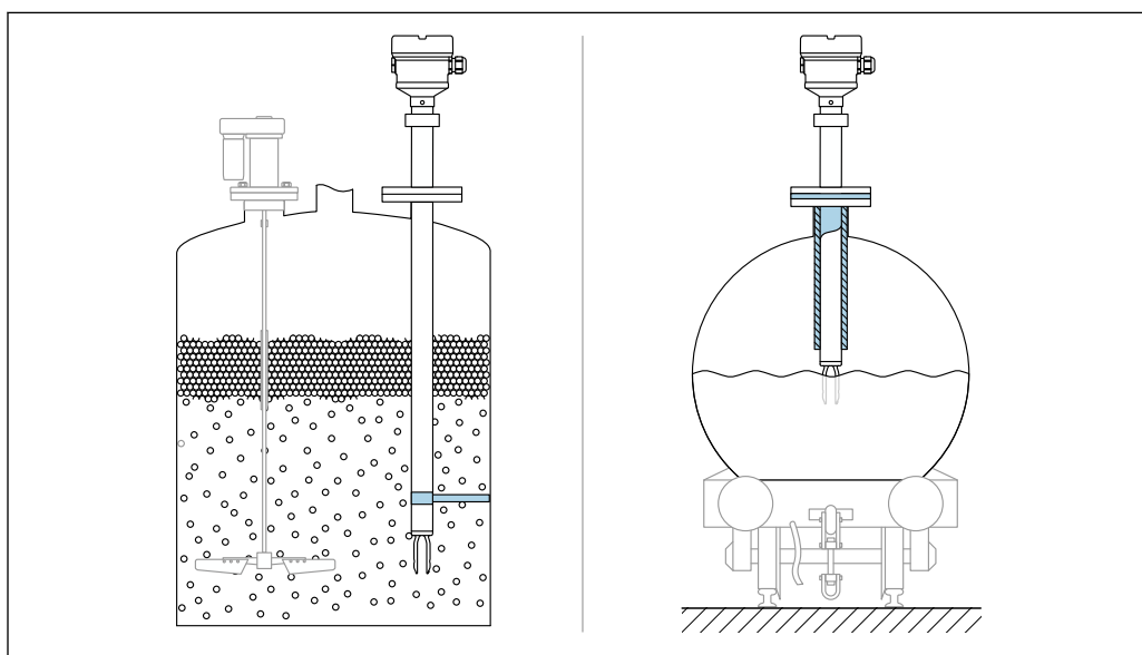
15 Примеры использования опоры при динамической нагрузке
