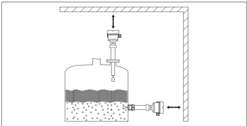
11 Учет необходимого свободного пространства
