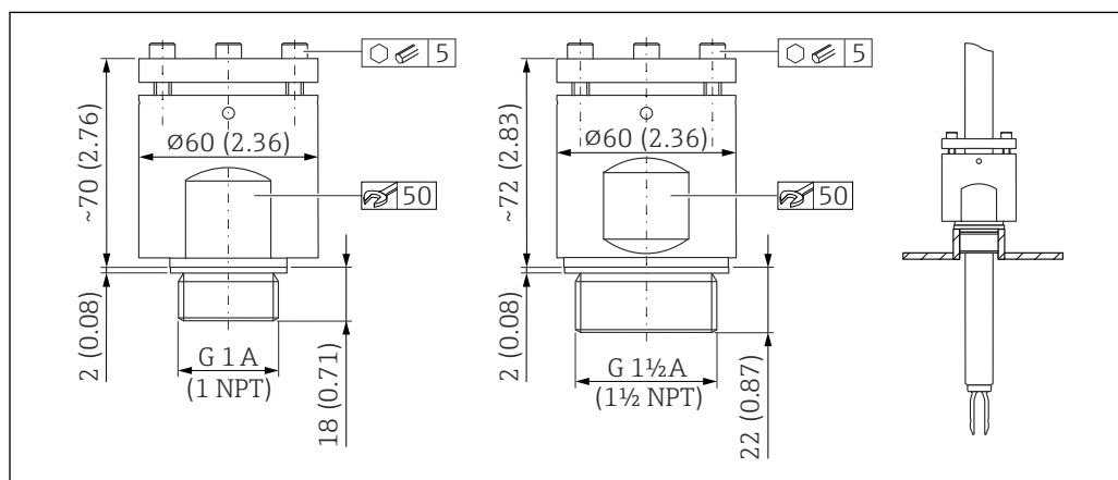
i 36 Скользящие муфты для использования в условиях высокого давления. Единица измерения мм (дюйм)
