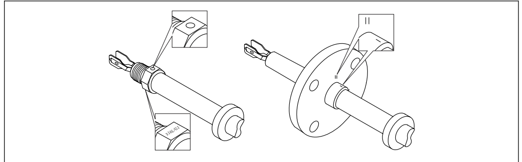
12 Маркировка для выравнивания вибрационной вилки
