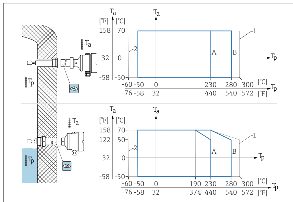
16 Зависимость допустимой температуры окружающей среды T_a в зоне корпуса от рабочей температуры T_p в резервуаре
