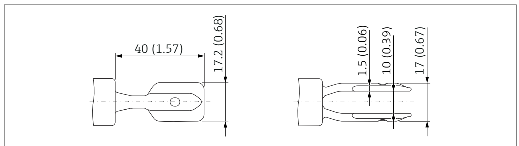
21 Вибрационная вилка. Единица измерения мм (дюйм)
