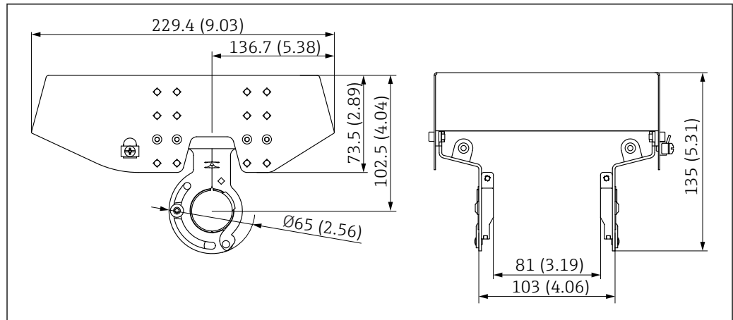
31 Защитный козырек от погодных явлений для корпуса с двумя отсеками. Единица измерения мм (дюйм)
