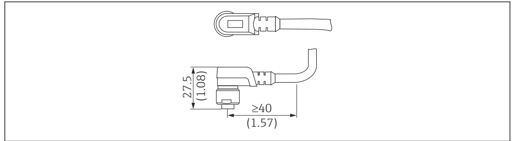
34 Штепсельный разъем M12 IP67. Единица измерения мм (дюйм)
