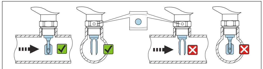
13 Монтаж в трубопроводах (следует учитывать положение вилки и маркировку)
