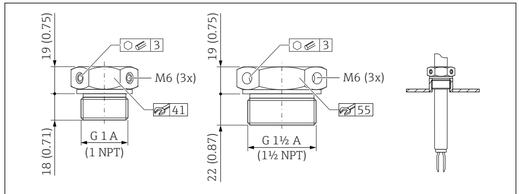
35 Скользящие муфты для работы при отсутствии давления, p_e = 0 бар (0 фунт/кв. дюйм). Единица измерения мм (дюйм)
