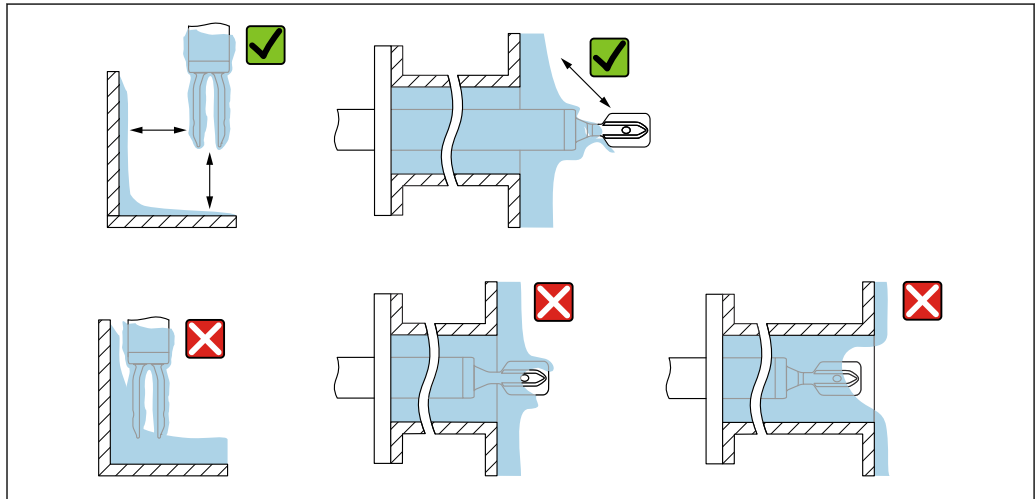
10 Примеры монтажа в технологической среде с высокой вязкостью
