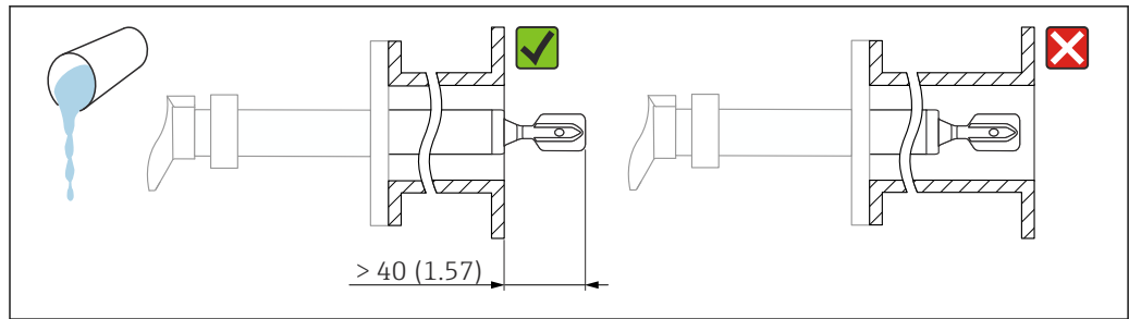
9 Пример монтажа для жидкостей с высокой вязкостью. Единица измерения мм (дюйм)
