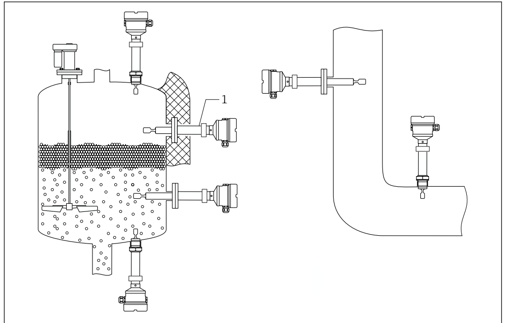
7 Примеры монтажа в резервуаре, баке или трубопроводе
