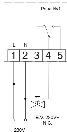
Рис. 2 Схема подключения к нормально закрытому клапану
