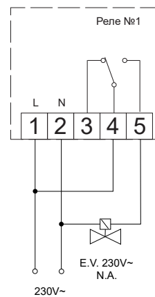
Рис. 3 Схема подключения к нормально открытому клапану
