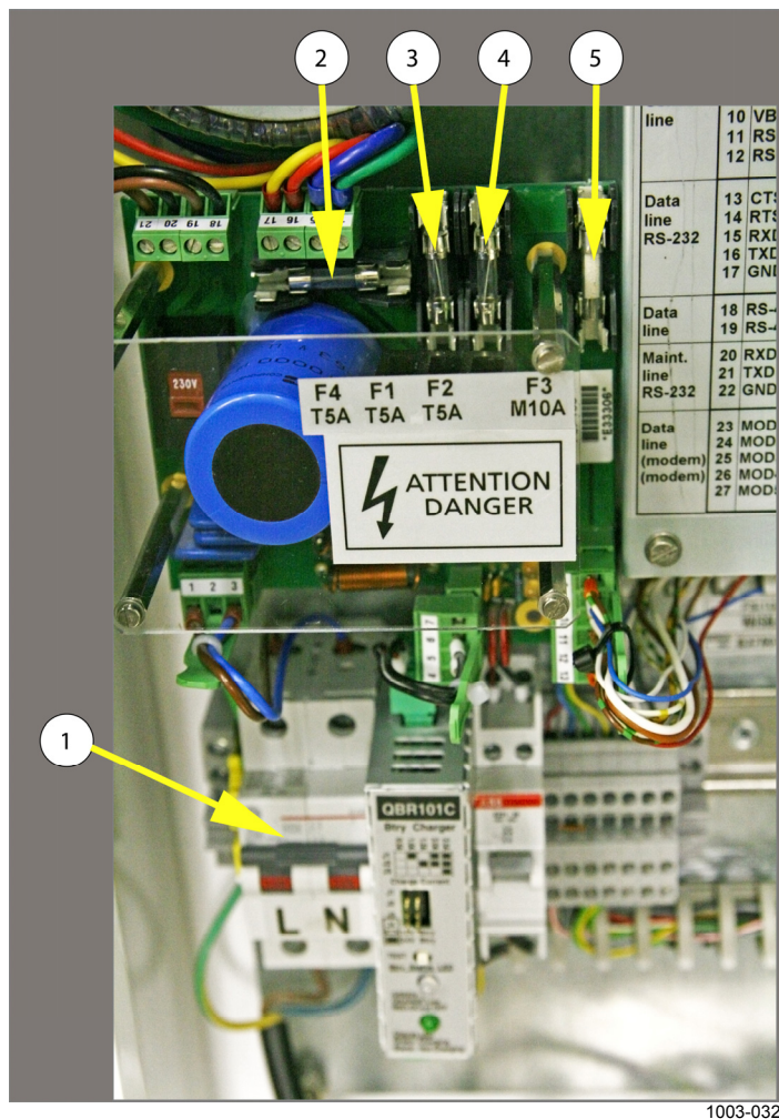
Рис. 53. Расположение предохранителей на плате FSP103.
