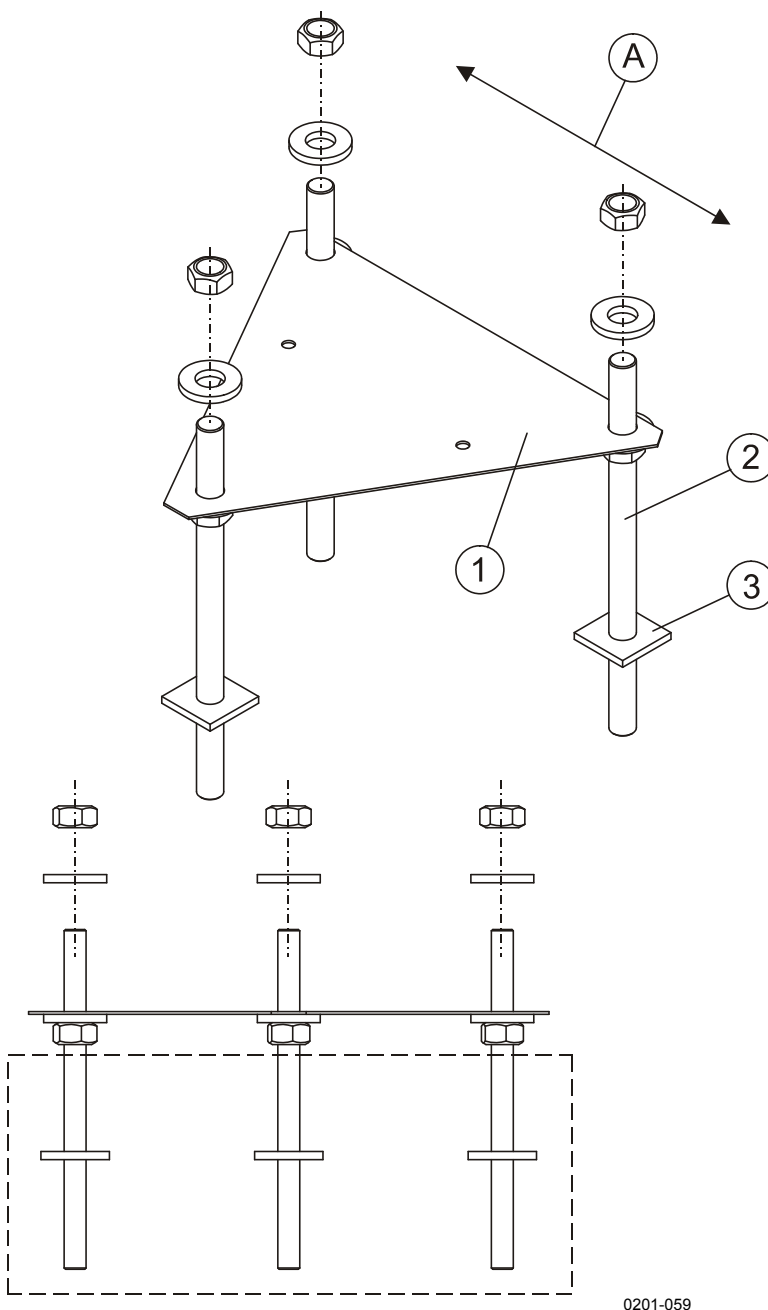
Рис. 6. Возведение фундамента для FS11
