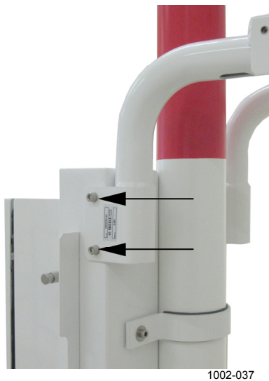
Рис. 11. Закрепление плеча датчика установочными винтами.
