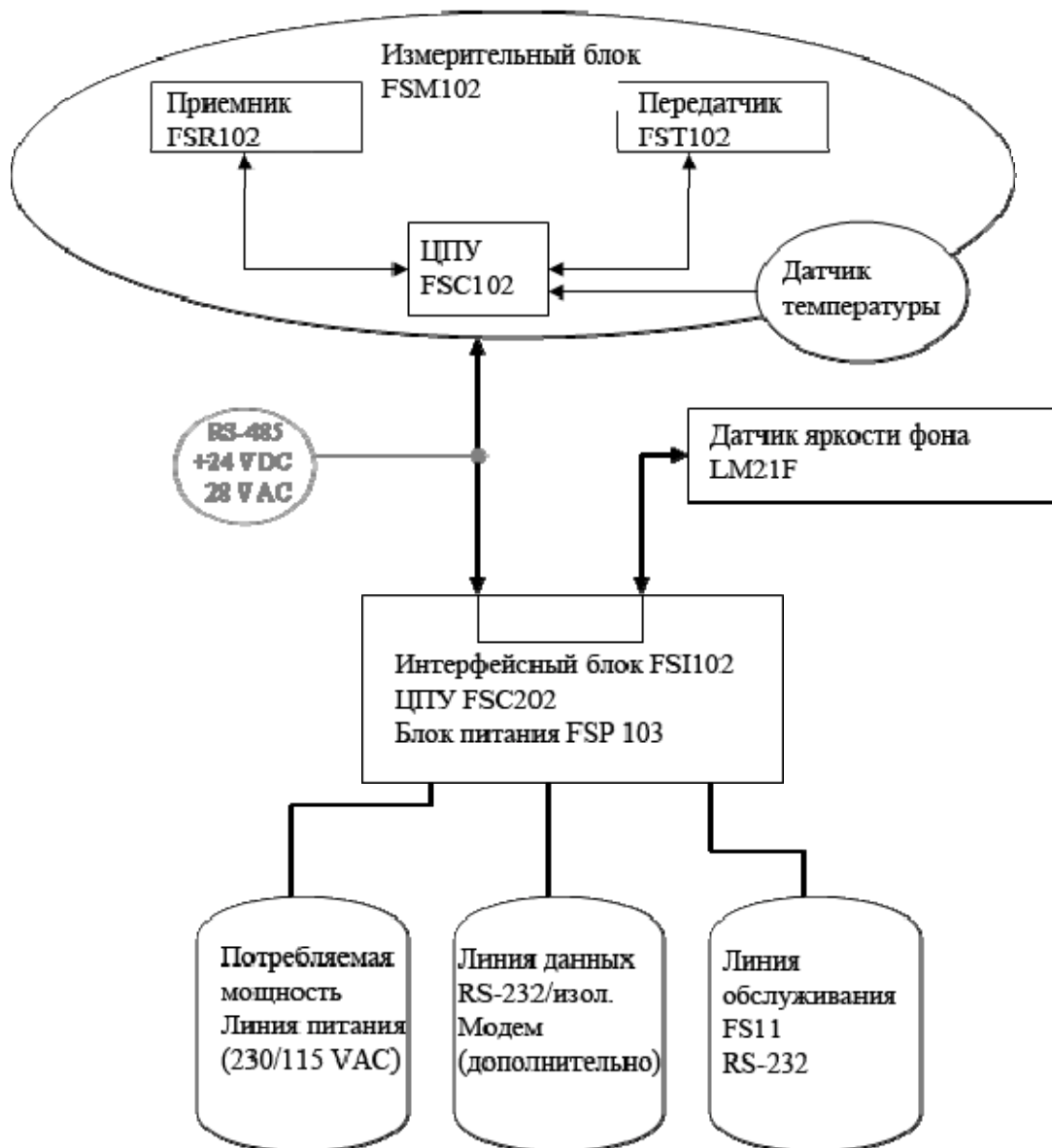
Рис. 35. Блок-схема датчика FS11
