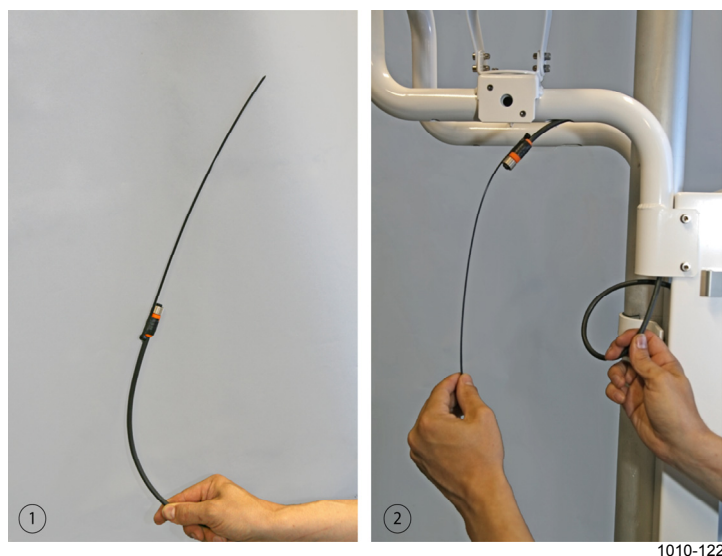
Рис. 16. Протяжка кабельного разъема с помощью веревки
