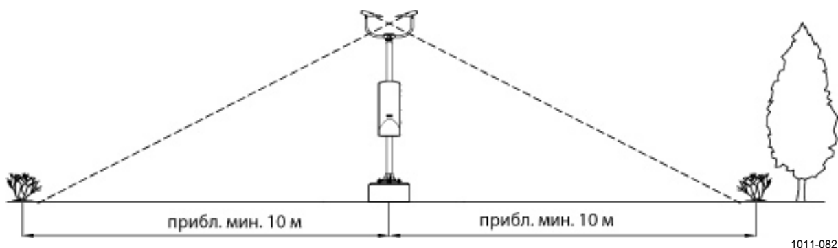
Рис. 2. Рекомендуемое расположение датчика видимости FS11 с мачтой FSAM250/FSFM250
