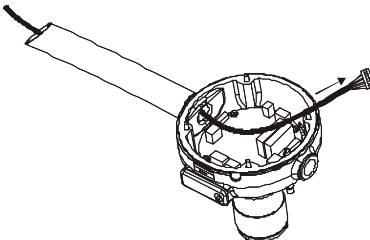
Рис. 50. Вытягивание контрольного кабеля из трубы корпуса
