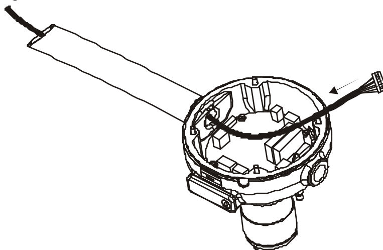
Рис. 48. Вытаскивание контрольного кабеля в оптическую головку
