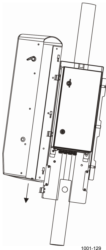
Рис. 21. Монтаж радиационного экрана
