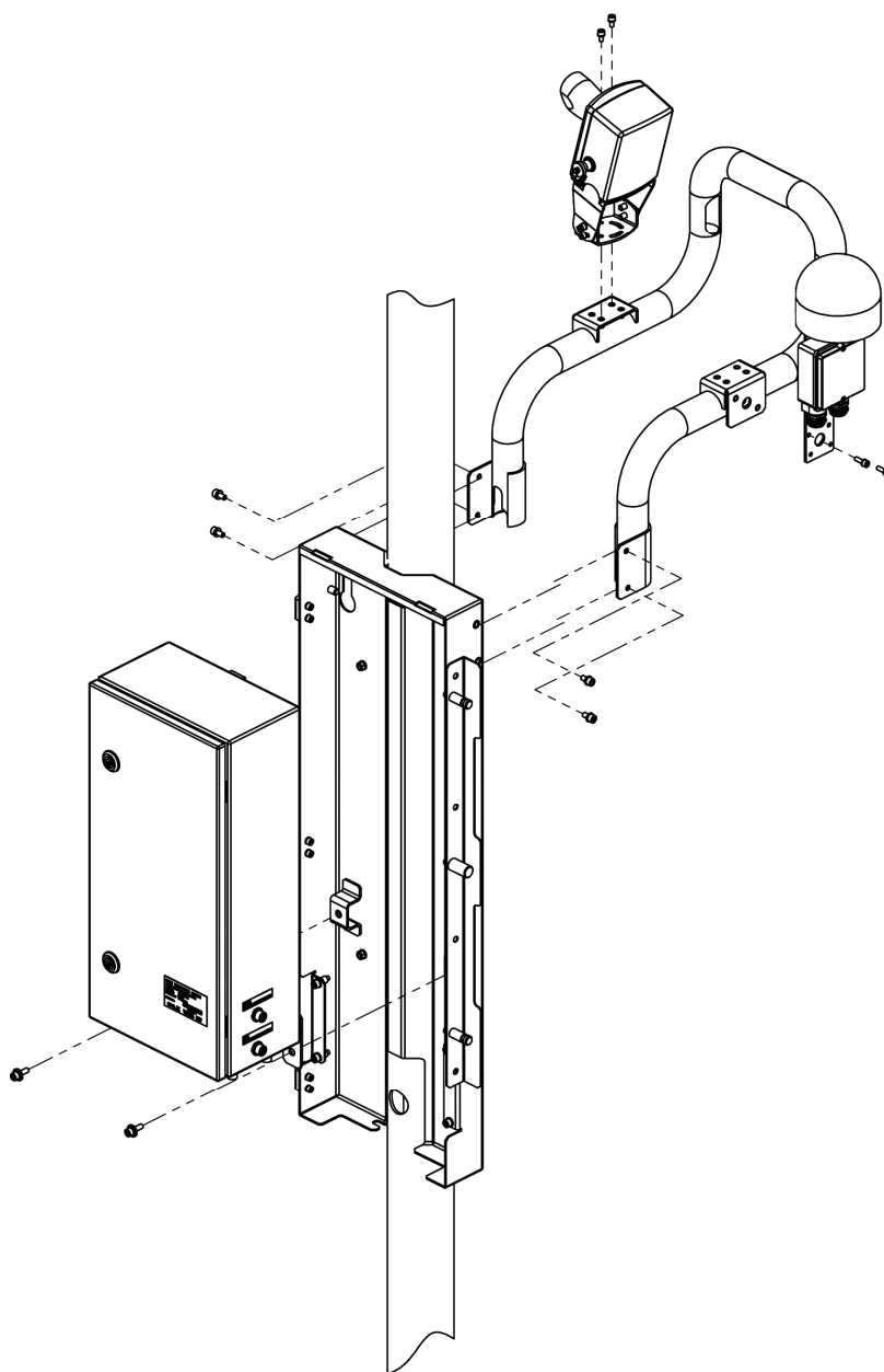
Рис. 20. Сборка плеча датчика
