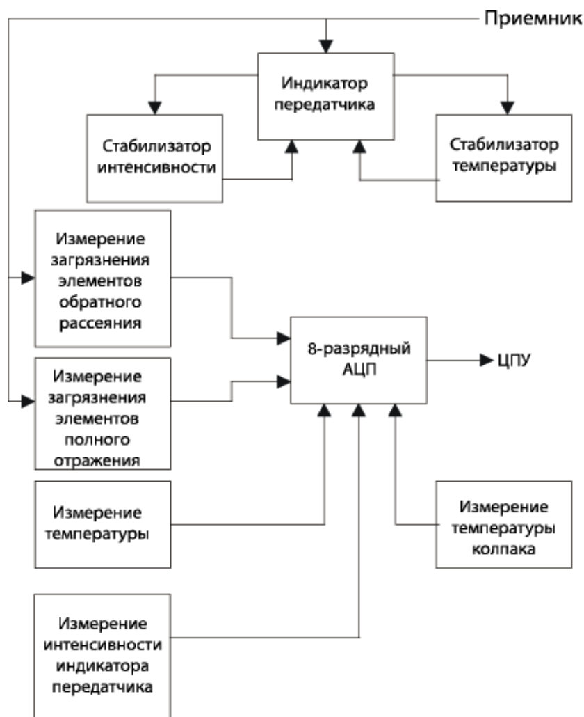
Рис. 36. Блок-схема передатчика FST102
