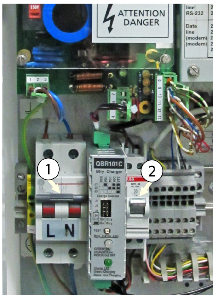
Рис. 34. Включение блока
