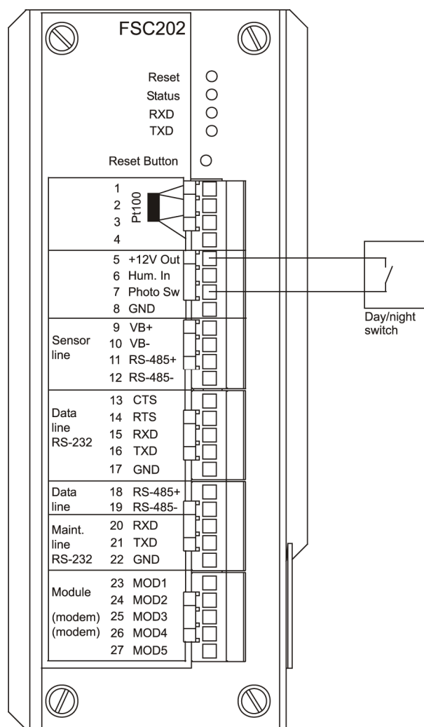
Рис. 32. Подключение фотопереклювателя день/ночь
