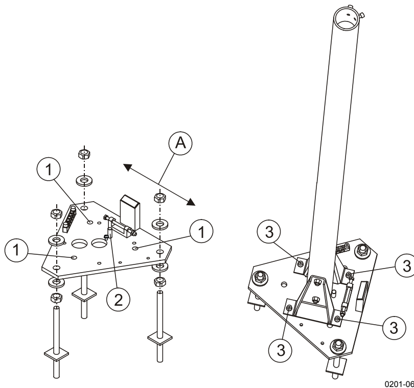
Рис. 10. Установка алюминиевой мачты FS11 с помощью монтажного комплекта FS211296
