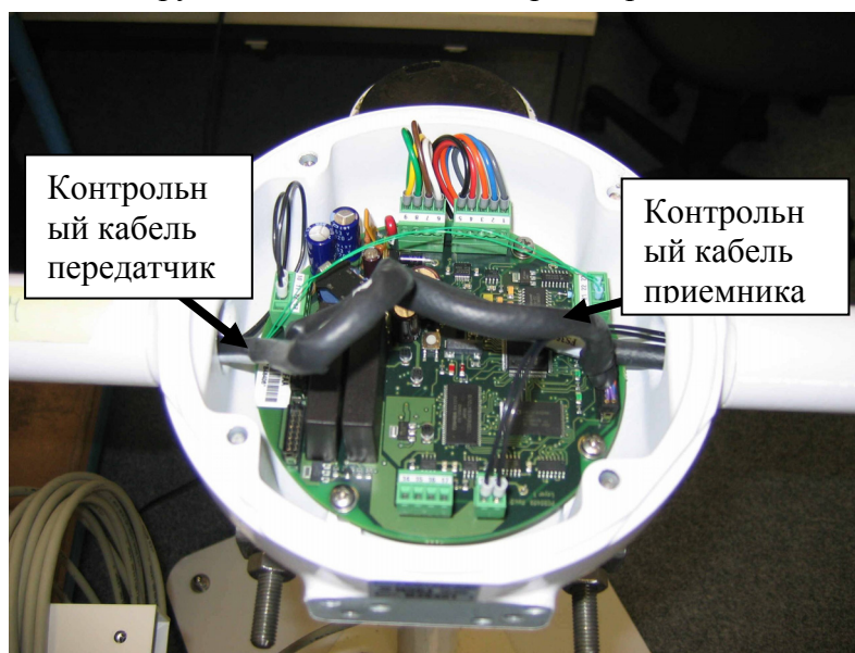
Рис. 45. Контрольные кабели передатчика и приемника датчика видимости
