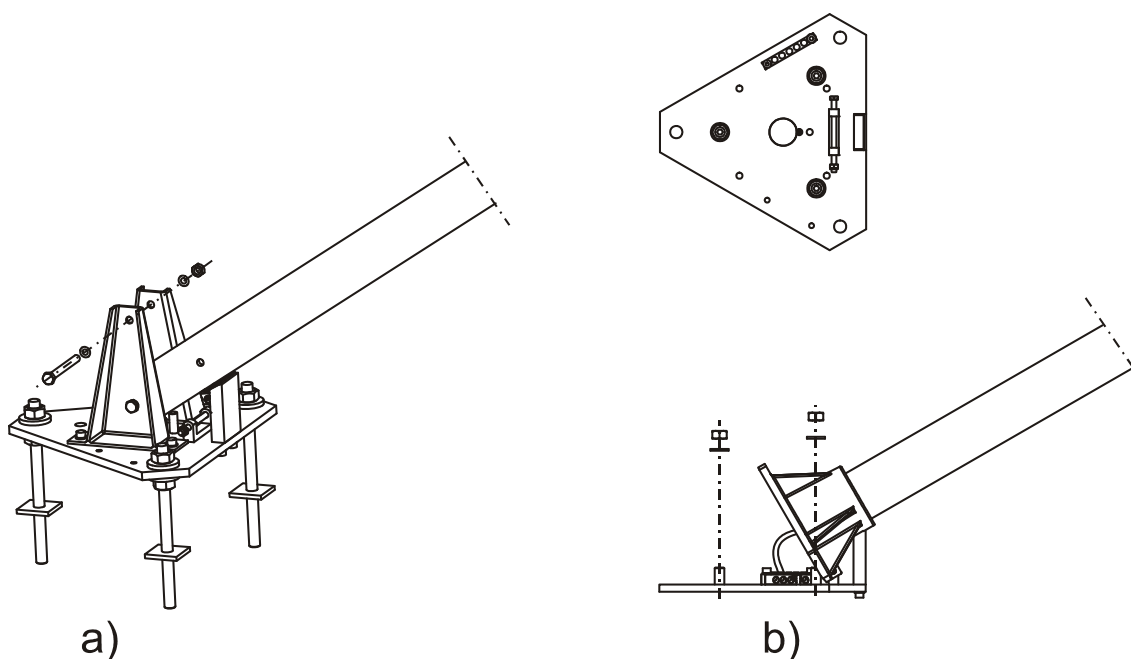
Рис. 13. Наклон алюминиевой и хрупкой мачт
