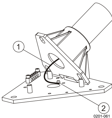
Рис. 9. Монтаж кабеля заземления хрупкой мачты FS11
