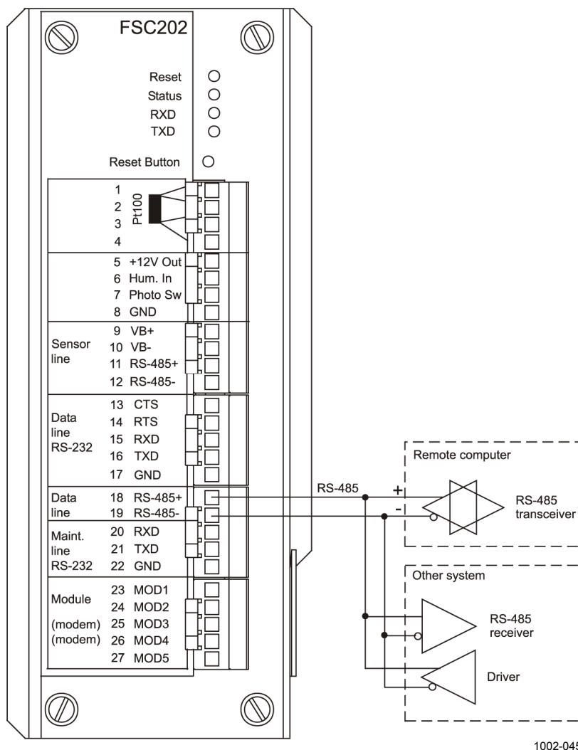
Рис. 27. Связь в стандарте RS-485
