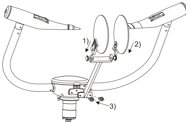
Рис. 41. Сборка и установка калибратора
