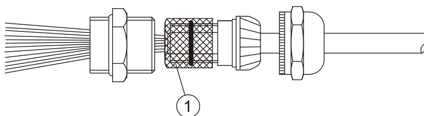
Рис. 25. Инструкция по заземлению кабеля
