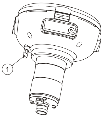
Рис. 39. Расположение датчика температуры поверхности
