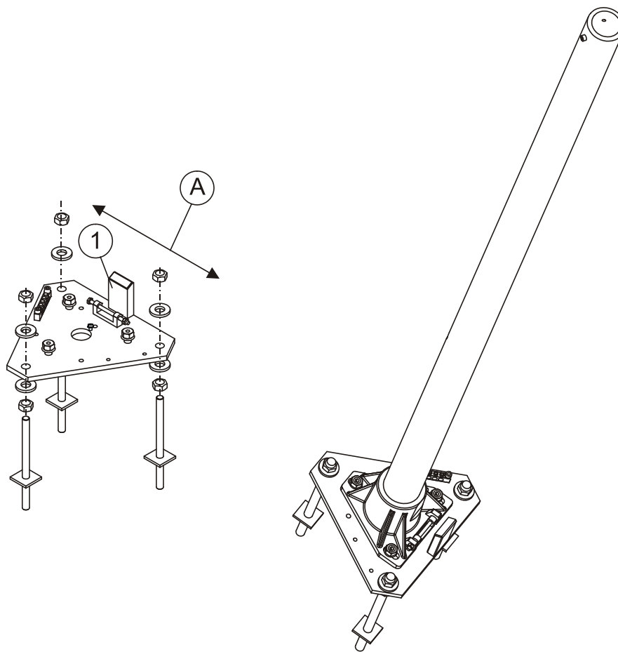
Рис. 8. Установка мачты FS11 с помощью монтажного комплекта FS211296
