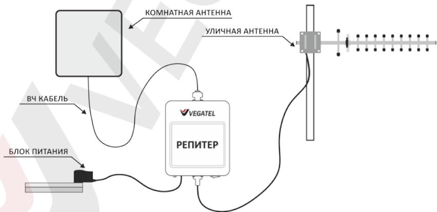
СХЕМА ПОДКЛЮЧЕНИЯ РЕПИТЕРА
