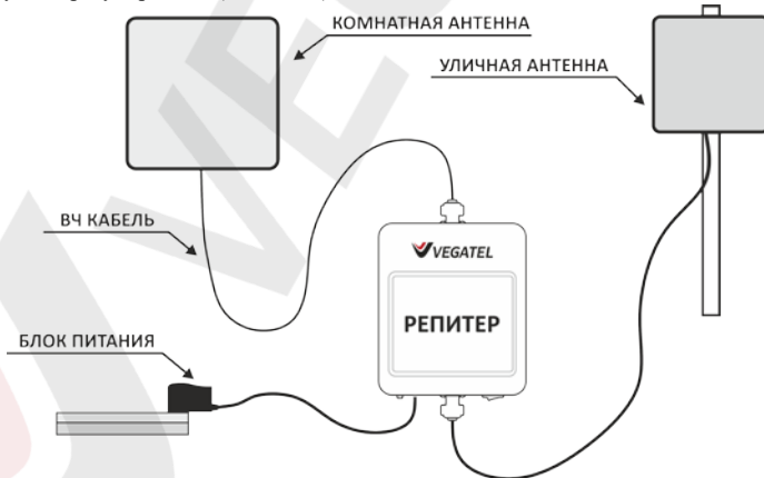
СХЕМА ПОДКЛЮЧЕНИЯ РЕПИТЕРА
