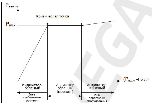
График изменения индикации «Перегрузка» в зависимости от мощности входящего сигнала
