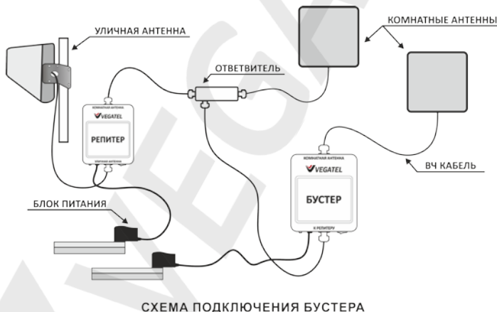
Рис.1. Схема подключения бустера
