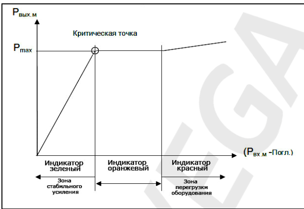
График изменения индикации Alarm в зависимости от мощности входящего сигнала
