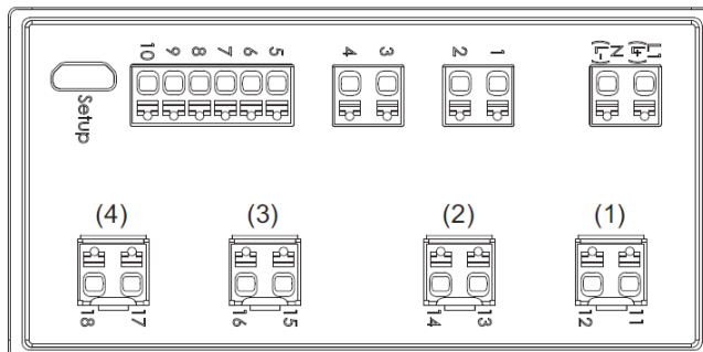
Тип 702114 (96 мм × 96 мм)
