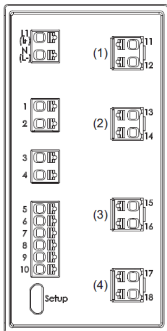
Тип 702112 (48 мм × 96 мм)
