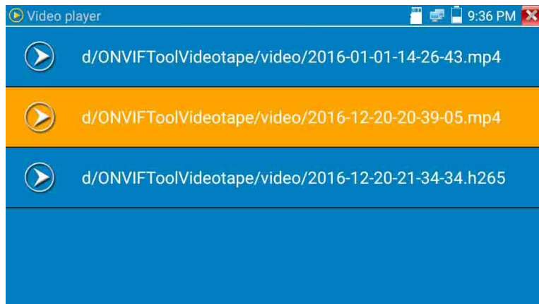
Рис. 48 Меню видеоплеера
