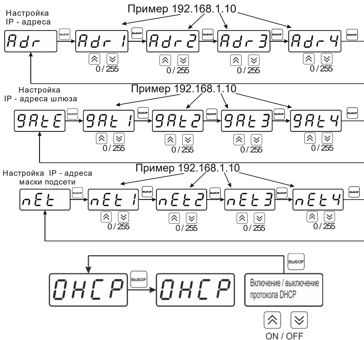
Рисунок 6.13 Сетевые настройки
