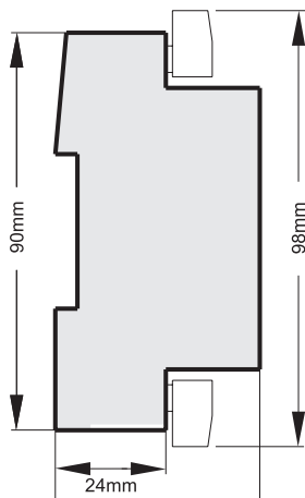
Вид сбоку
