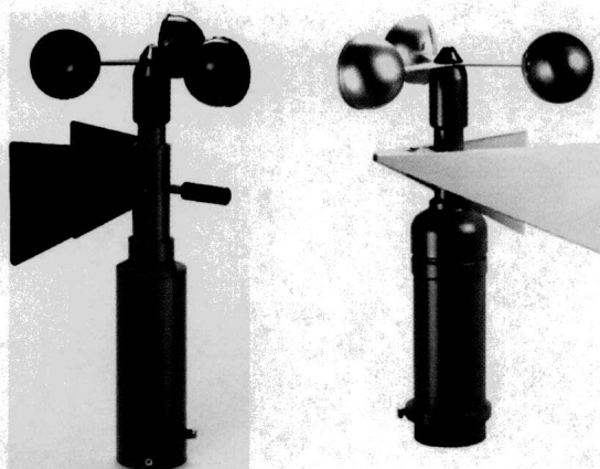
Рисунок 10 – Общий вид анеморумбометров МПВ-502.14513 (Два вида исполнения)
