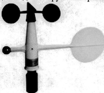
Рисунок 13 – Общий вид анеморумбометров МПВ-502.14516
