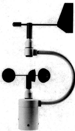
Рисунок 12 – Общий вид анеморумбометров МПВ-502.14581
