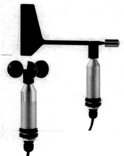
Рисунок 3 – Общий вид анеморумбометров МПВ-602.14564
