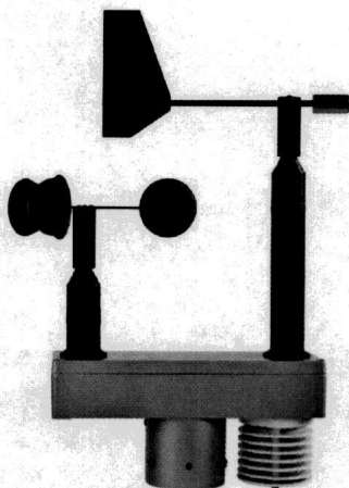
Рисунок 13 – Общий вид анеморумбометров МПВ-502.14516
