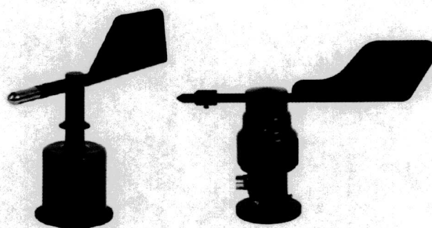
Рисунок 9 – Общий вид анеморумбометров МПВ-602.12100.2 (Два вида исполнения)
