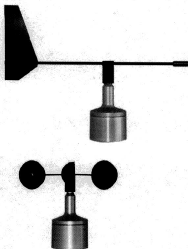
Рисунок 6 – Общий вид анеморумбометров МПВ-602.14566
