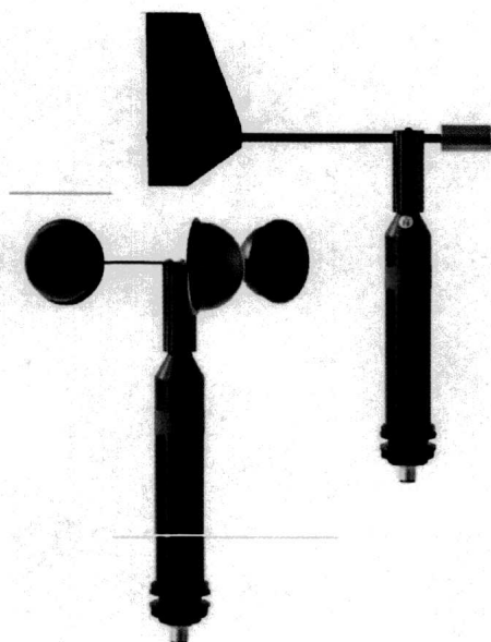
Рисунок 7 – Общий вид анеморумбометров МПВ-602.14521
