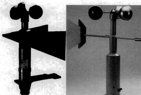
Рисунок 11 – Общий вид анеморумбометров МПВ-502.14530 (Два вида исполнения)
