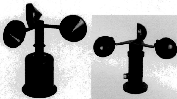
Рисунок 8 – Общий вид анеморумбометров МПВ-602.12100.1 (Два вида исполнения)
