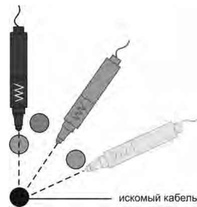
Рисунок 5.4.2 – Отбор жилы по минимуму сигнала
