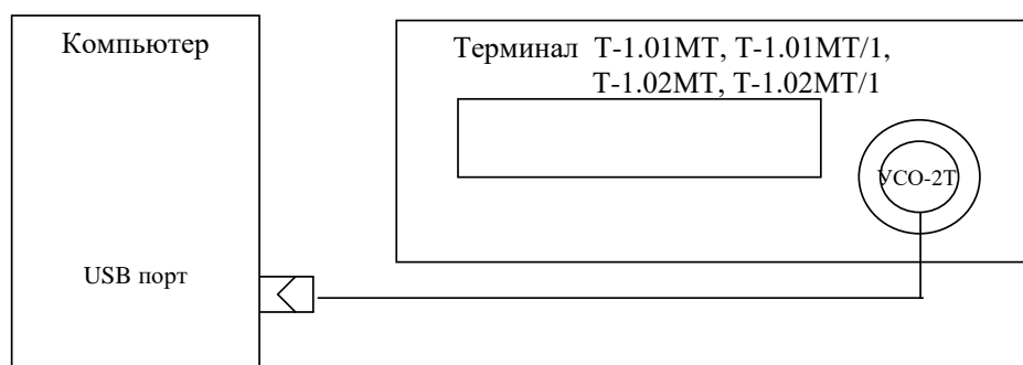
Рисунок 3 - Схема подключения терминала к компьютеру через оптопорт УСО-2Т
