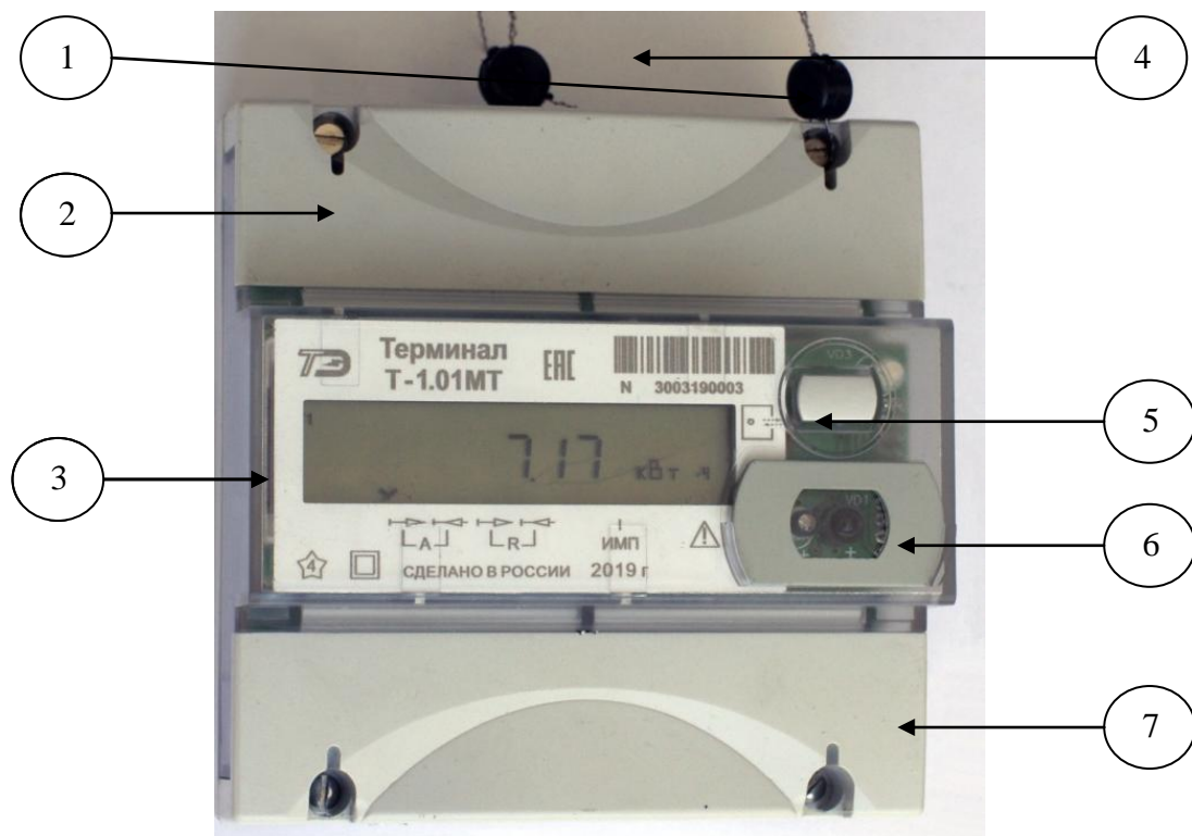
Рисунок 1 – Внешний вид терминала Т-1.01МТ
