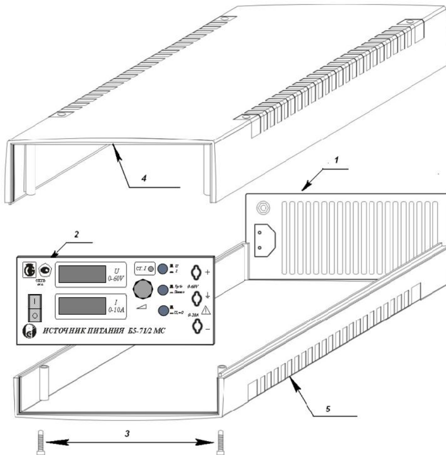
Рисунок 1.3 - Элементы корпуса источника питания.
