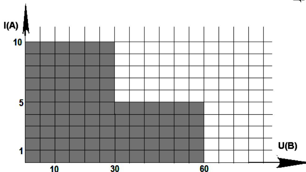
Рисунок 1.1 - Режимы установки выходных напряжения и тока
