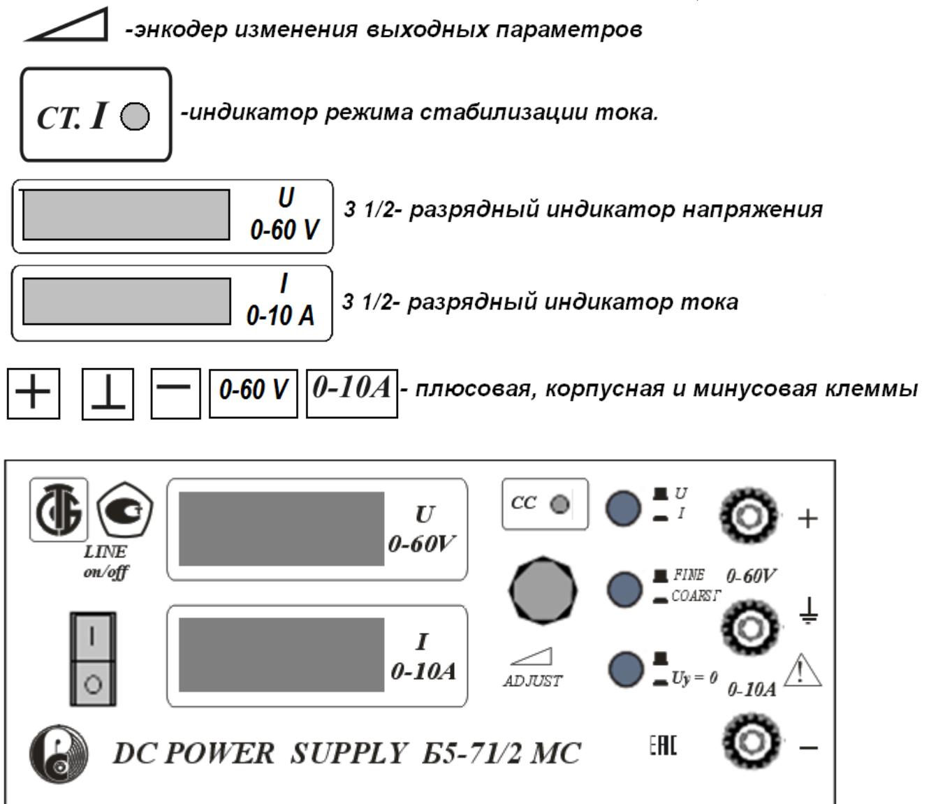
Рисунок 1.4 – Органы управления на передней панели источника питания
