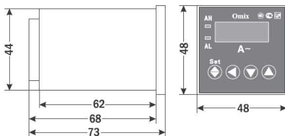
Рис. 3 – Размеры. Тип корпуса P44
