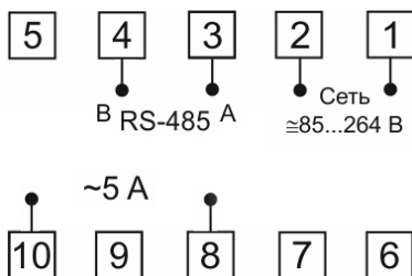
Рис. 7 – Схема подключения Тип корпуса P94, P99
