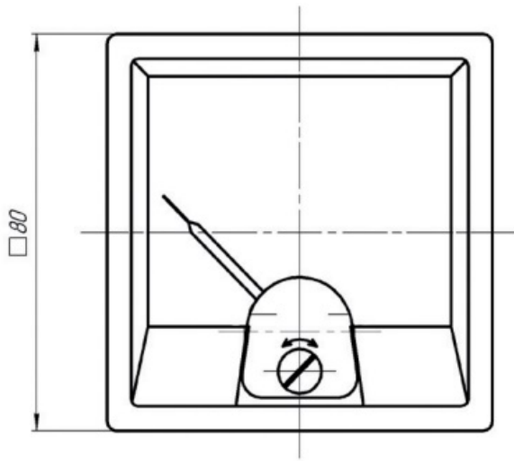
Габаритный чертеж Ц42307.
