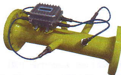
б) счетчик с ВС модификация 636128.310
