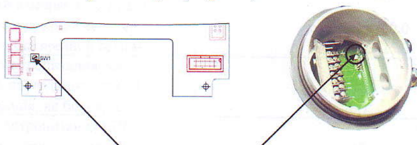
Расположение на плате БЭ переключателя защиты конфигурации счетчика от перезаписи
