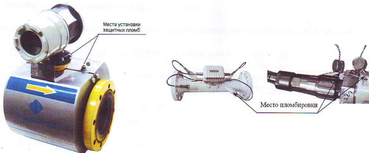
Рисунок 3 – Места пломбирования счетчика
