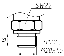
M20x1,5; G1/2" DIN 3852
