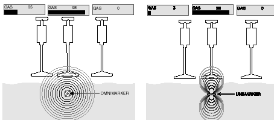
Рис. 32. Сигнал маркера Omni Marker Рис. 33. Сигнал маркера Uni Marker
