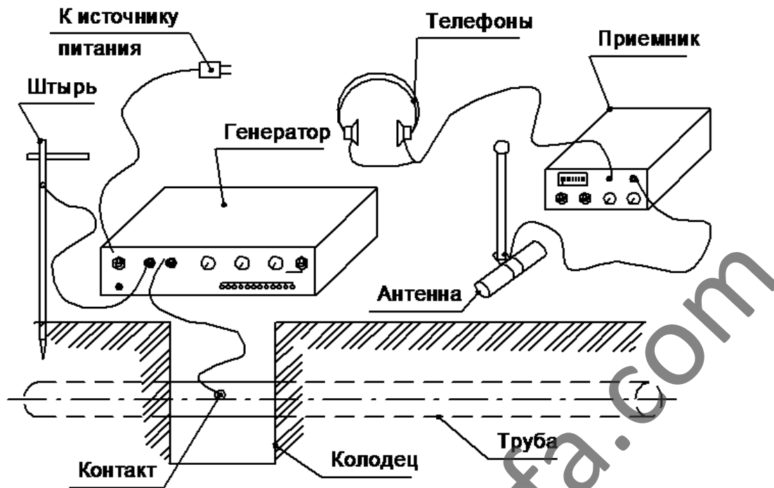
Рис.2. Функциональная схема активного режима искателя.
