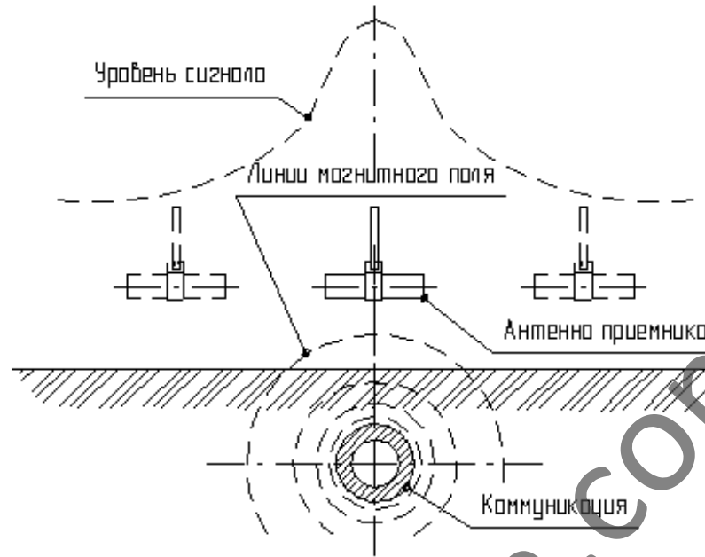
Рис.3. Схема поиска по максимуму сигнала.
