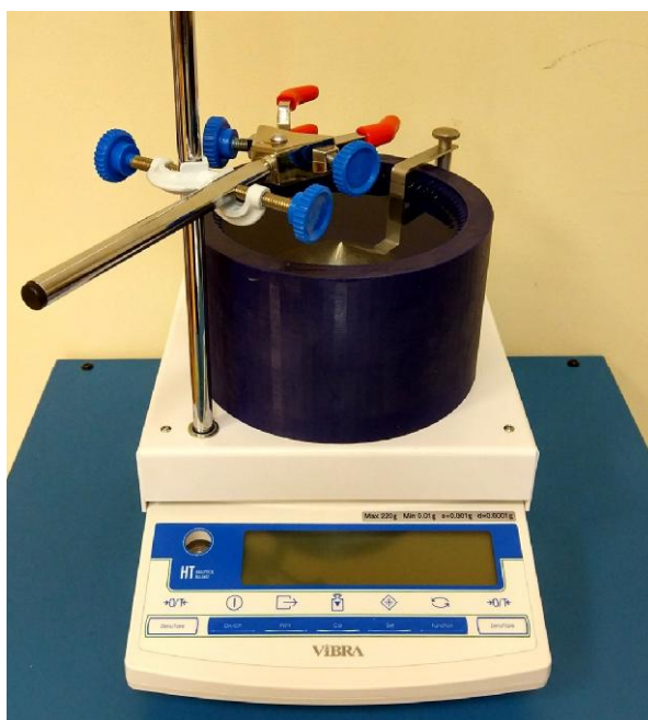
Рисунок 1 – Общий вид измерителя
