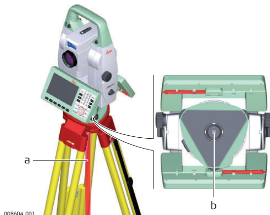
008604.001 а) Лазерный луч б) Выход лазерного луча
