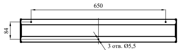
Установочные размеры светильника
