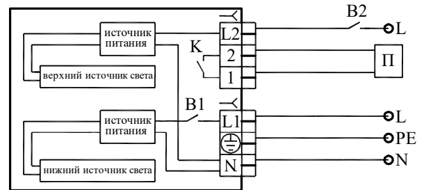
Схема электрическая подключения светильника.
