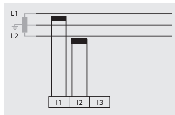
Рис. Показатели входа для измерения тока I3 приравниваются к нулю и не рассчитываются.
