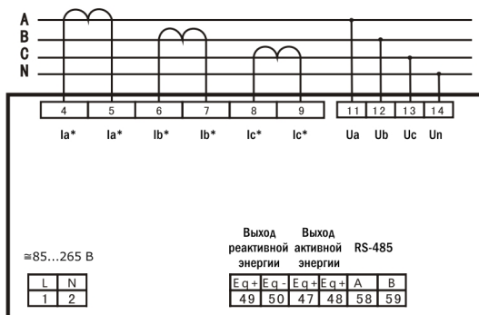
Рис. 3 – Клеммы подключения
