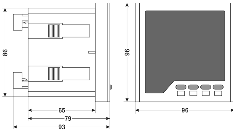
Рис. 2 – Размеры прибора
