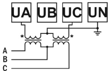
Рис. 4 – Подключение трансформатора напряжения (трехфазная цепь без нейтрали)
