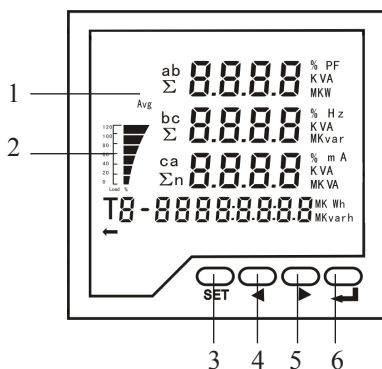
Рис. 1 – Управляющие элементы
